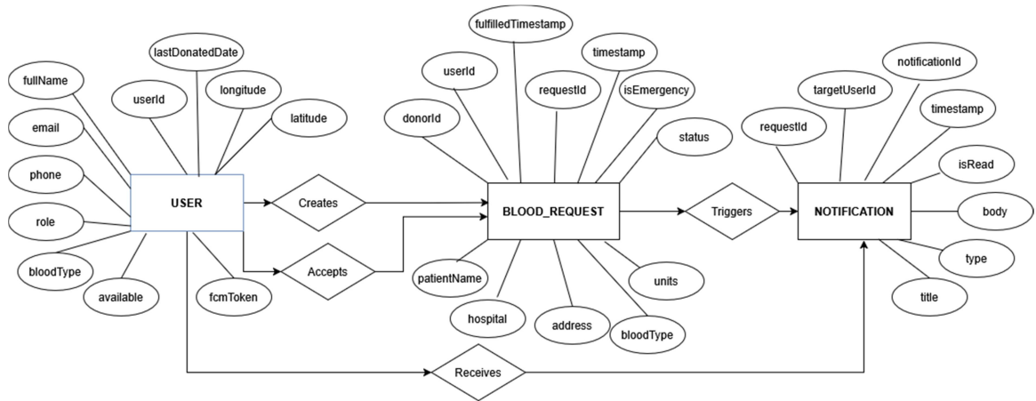
Figure 5 ER Diagram
