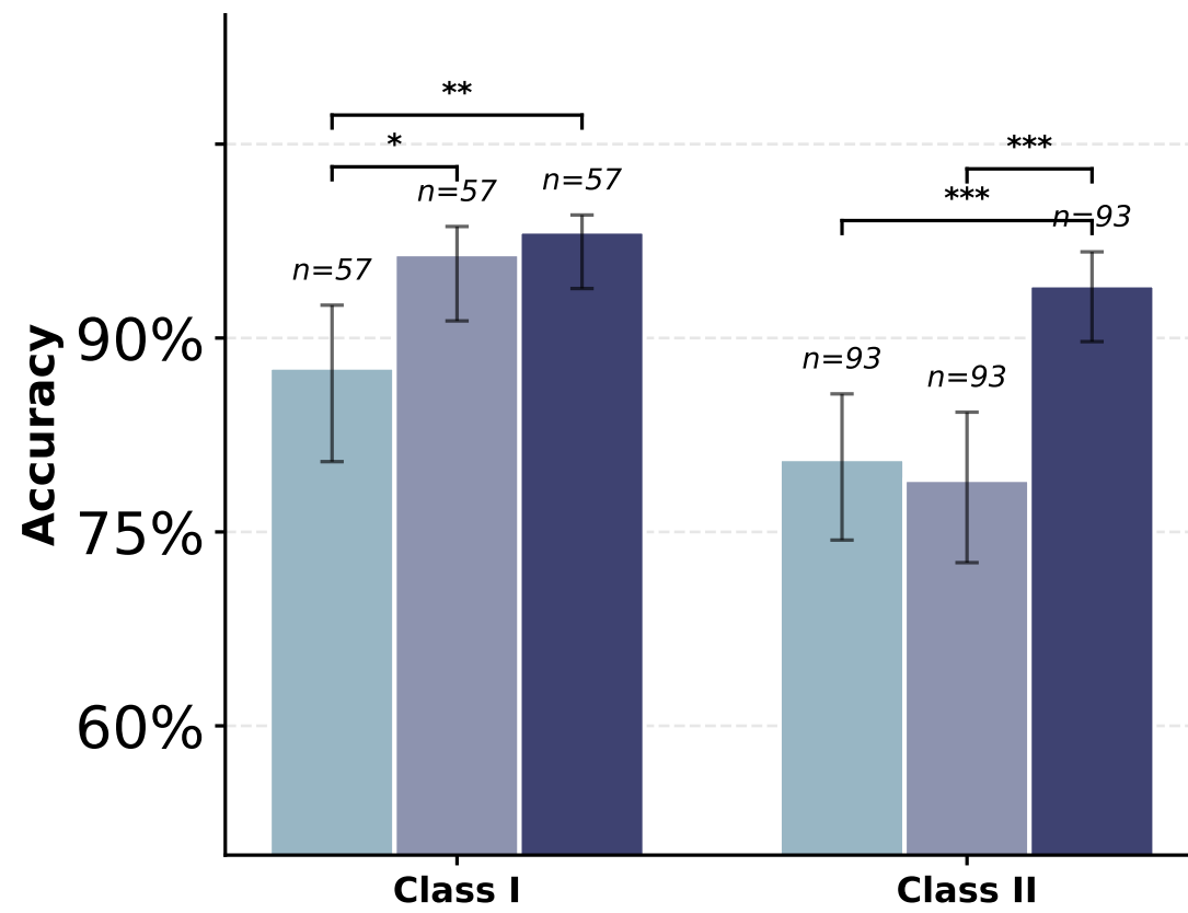
HGSVC CLR
