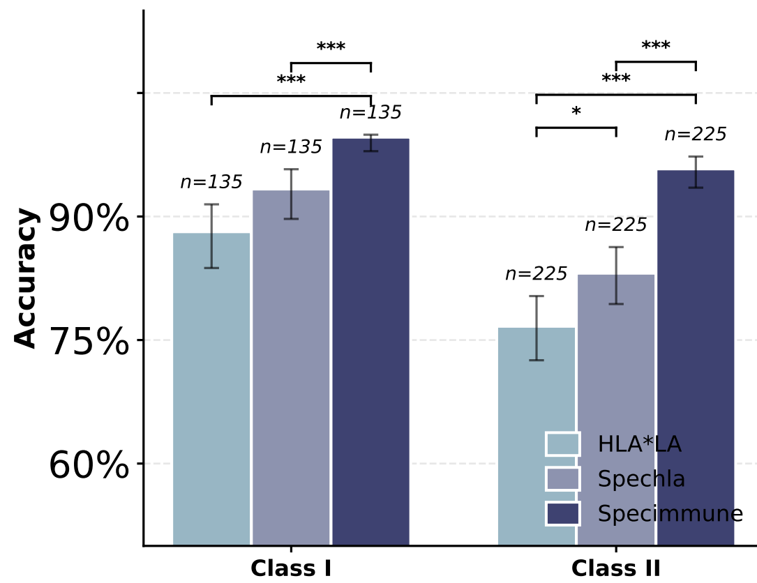
HPRC HiFi
