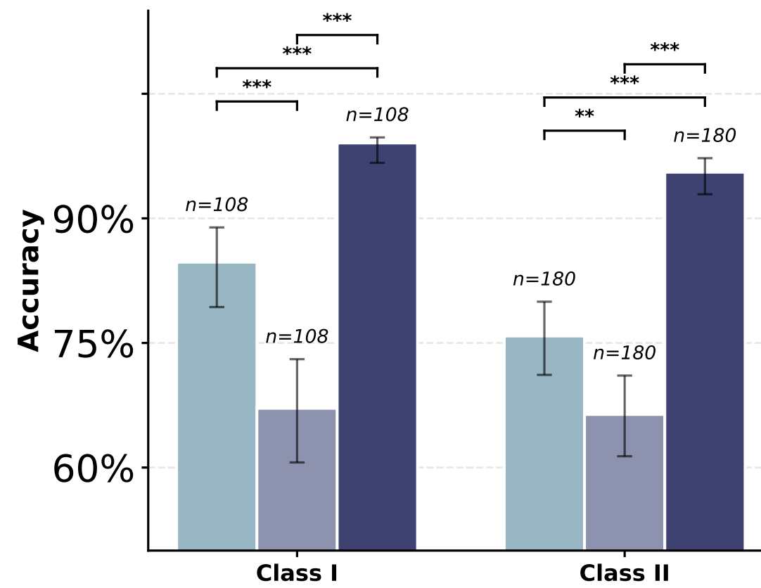
HPRC ONT
