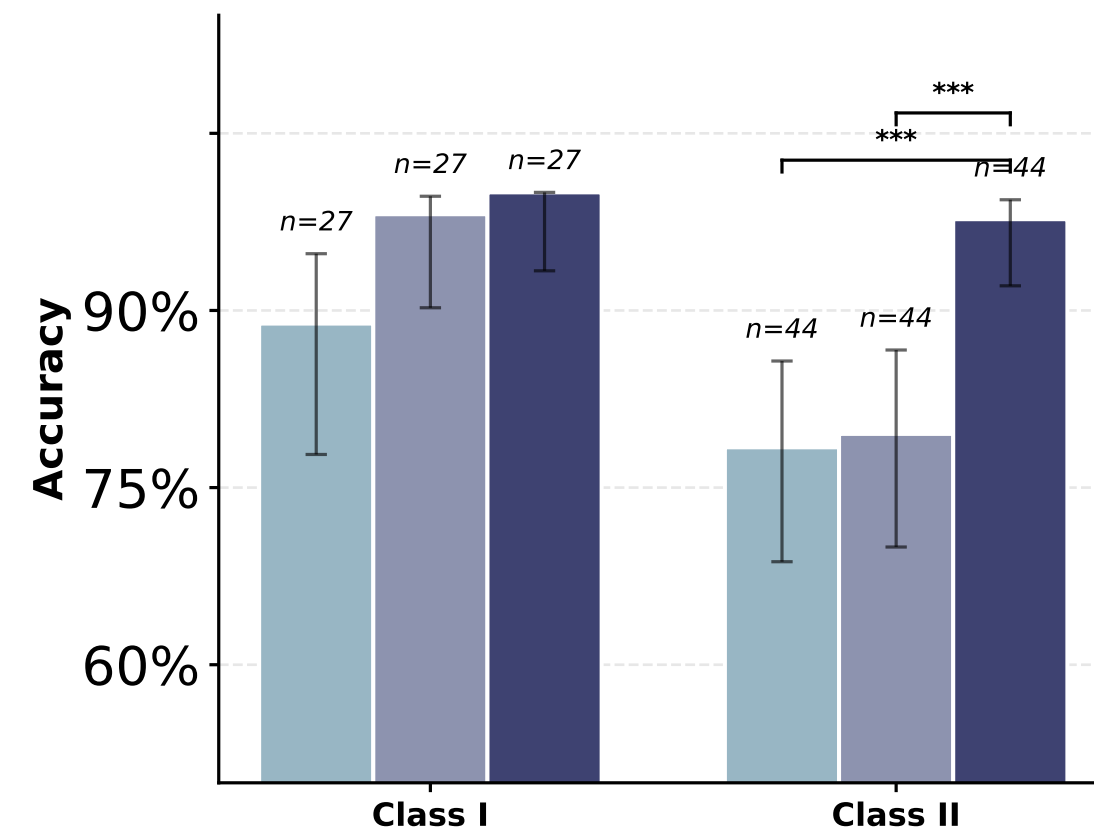
HGSVC HiFi
