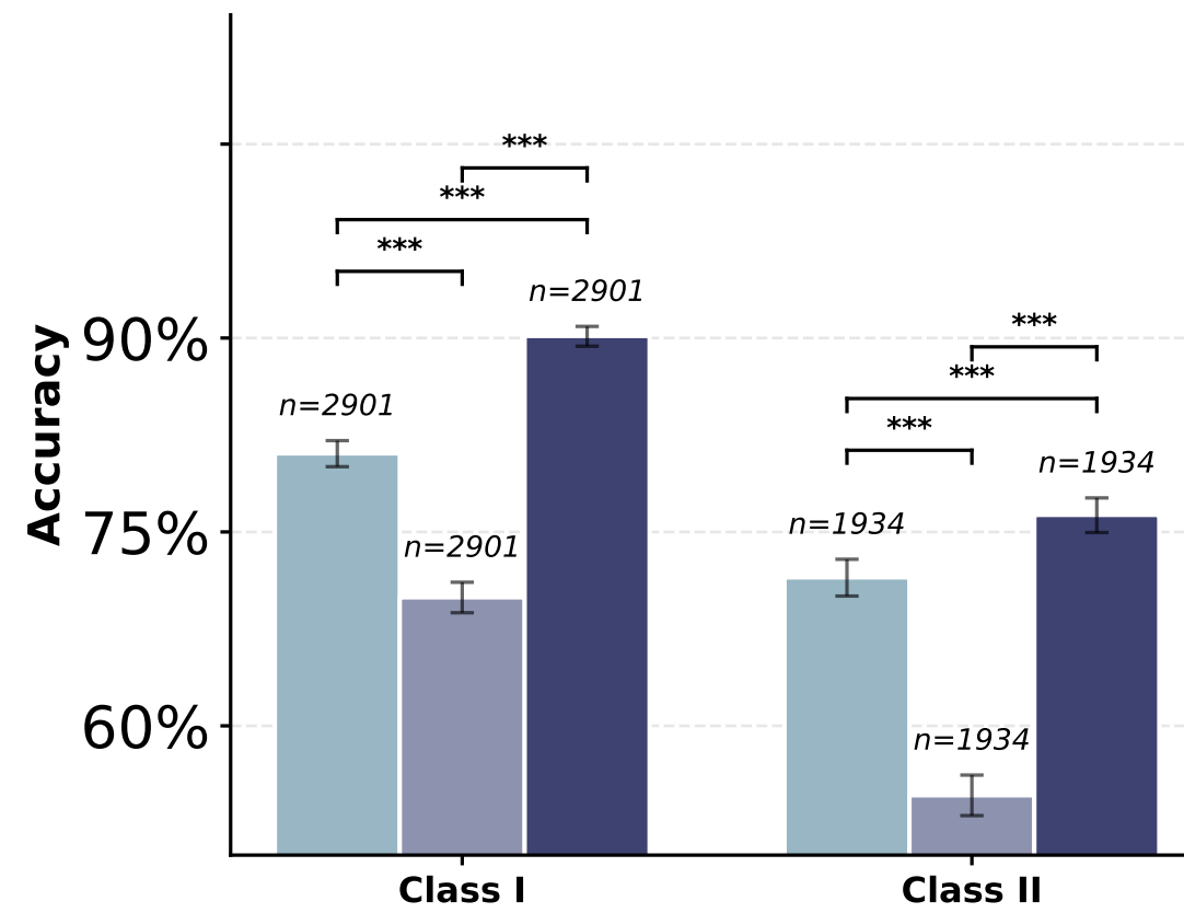
1KG ONT
