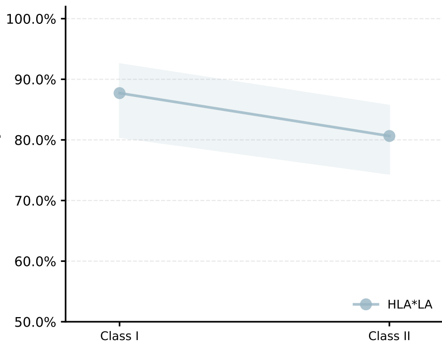
hprc_hifi
