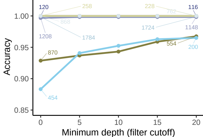
HPRC HiFi
