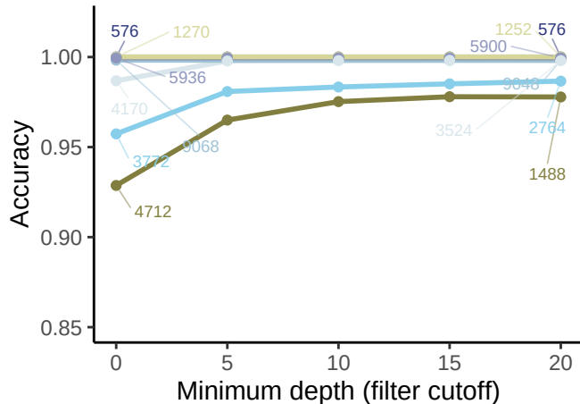
HPRC HiFi
