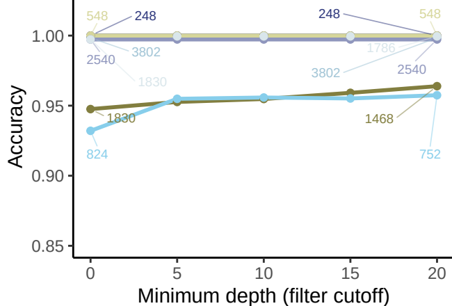
HPRC ONT
