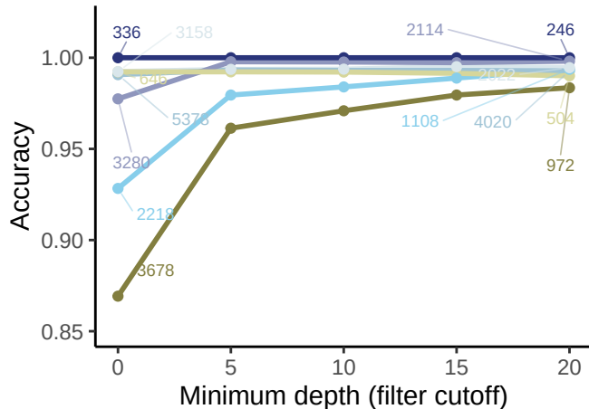
HPRC ONT
