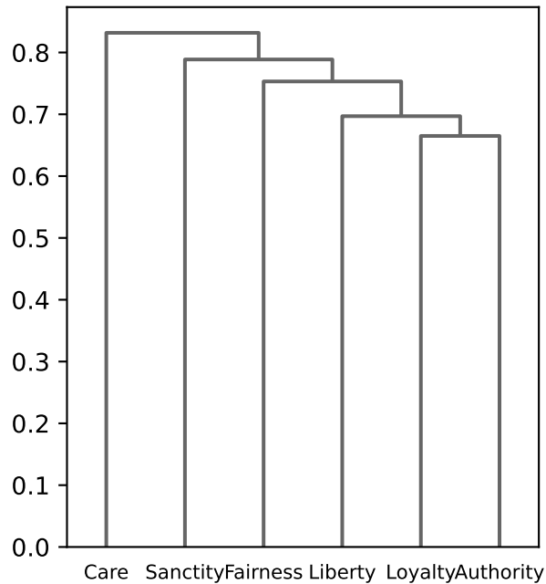
olmo3_sft_final (L16)
