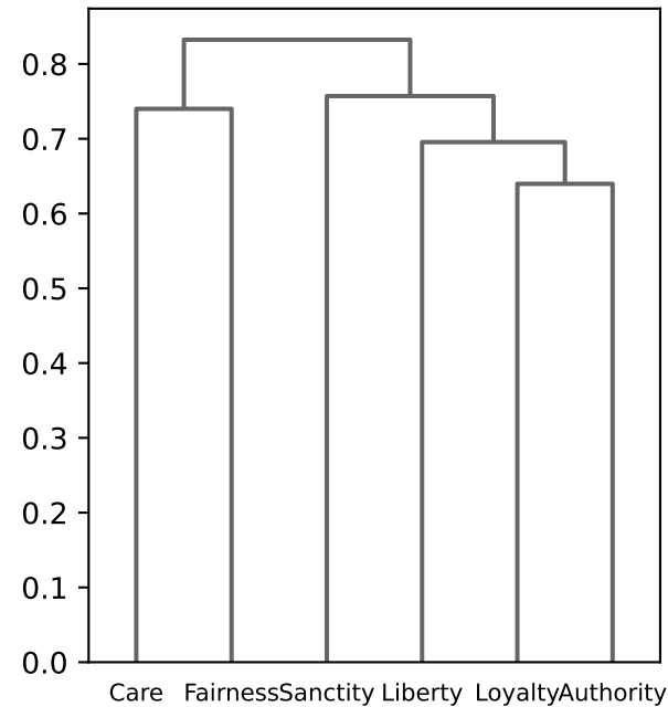
olmo3_base (L16)
