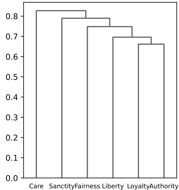
olmo3_dpo_final (L16)
