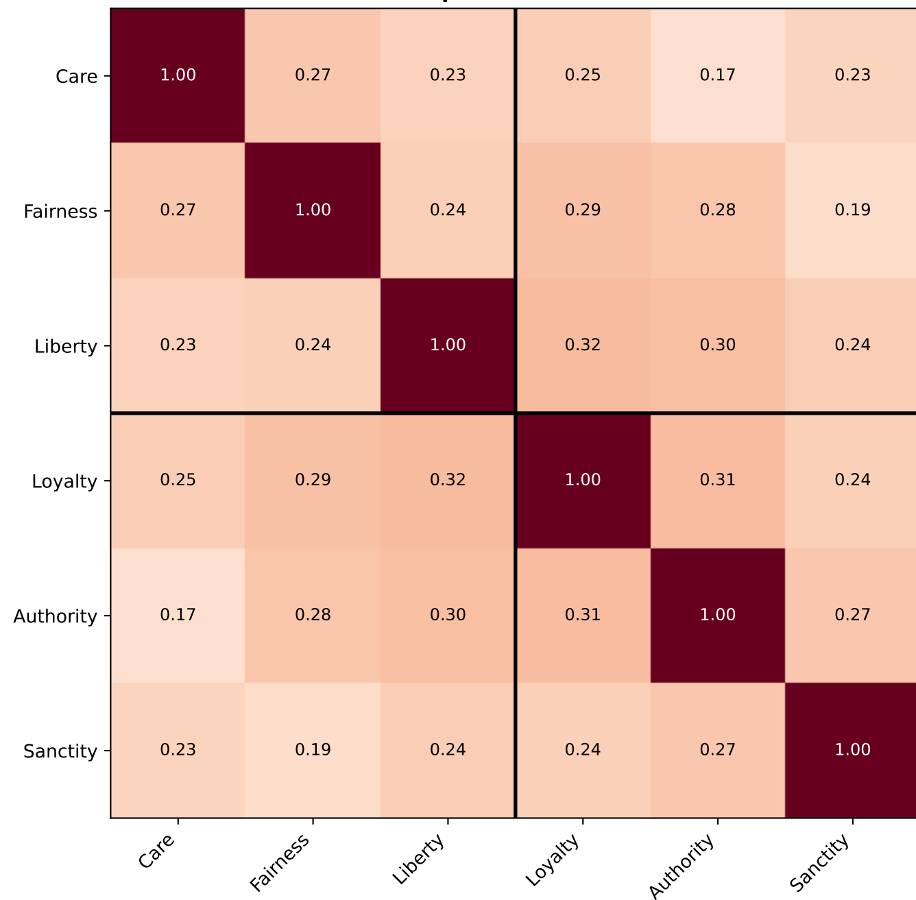
OLMo-2 1B (dense) Mean pairwise = 0.2548
