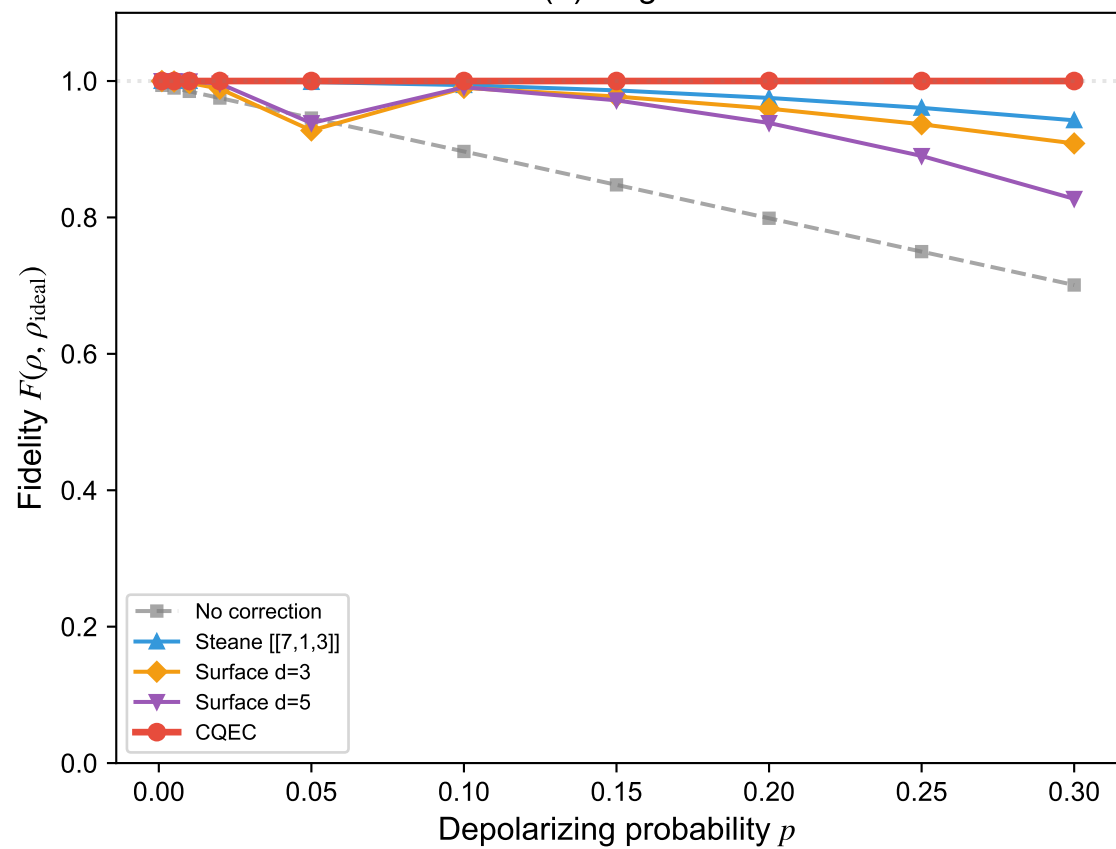
(d) Regev
