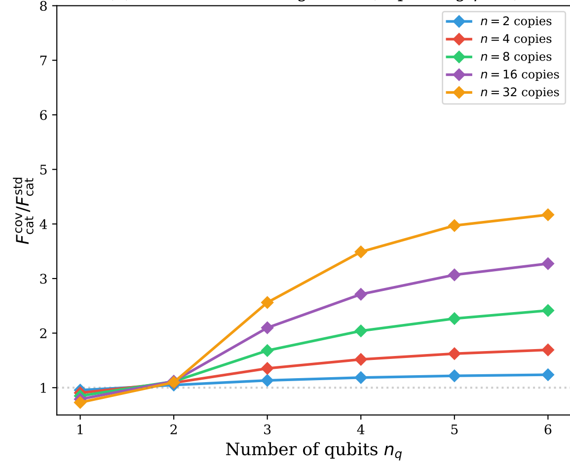
(d) Covariant advantage ratio (dephasing \gamma = 2 )
