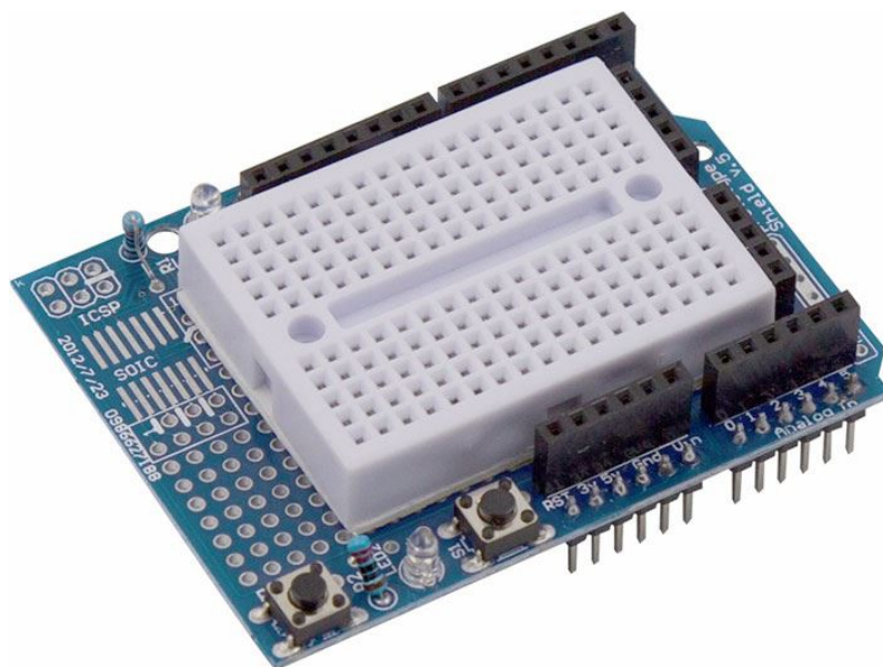
Obrázek 1.2: Prototypová vývojová deska s nepájivým polem pro testování obvodů
