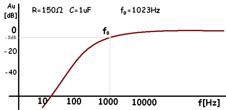
Obrázek 2.1: Amplitudová frekvenční charakteristika analogového RC filtru
