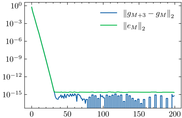
Erdős-Rényi graph
