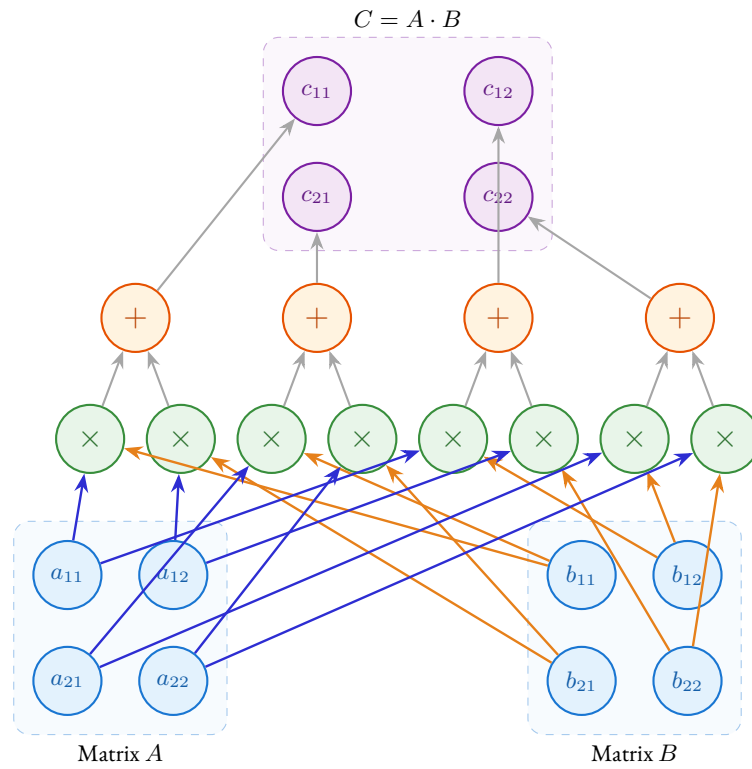
Figura 2.2: Circuito aritmetico per la moltiplicazione di matrici 2 \times 2 .
