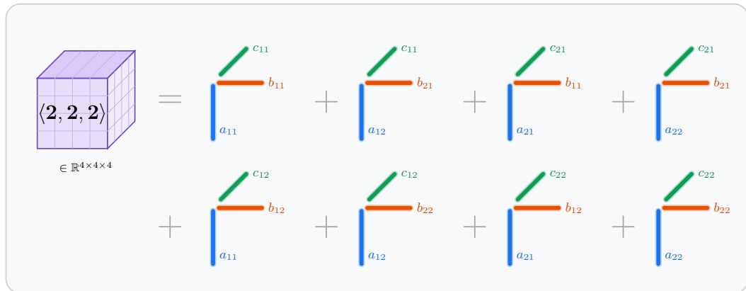
Figura 2.4: Decomposizione CP del tensore di moltiplicazione di matrici \langle 2, 2, 2 \rangle come somma di 8 tensori di rango uno.
