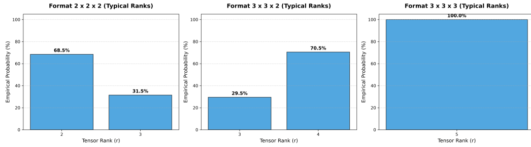
Figura 1.3: Distribuzione empirica dei ranghi per tensori casuali reali di formato 2 \times 2 \times 2 , 3 \times 3 \times 2 e 3 \times 3 \times 3 .
