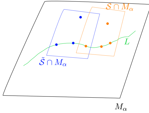
Figura 2.1: Interpretazione geometrica della costruzione nel caso k = 1 ( L è una retta, e gli M_{\alpha} sono piani). In questo caso L contiene almeno \mu \geq k + 1 = 2 punti di \tilde{\mathcal{S}} , e M_{\alpha} contiene almeno \mu + 1 \geq k + 2 = 3 di \tilde{\mathcal{S}} ; per ipotesi induttiva, 3 \leq \#(\tilde{\mathcal{S}} \cap M_{\alpha}) \leq \#(\mathcal{S} \cap M_{\alpha}) . A priori i punti di \mathcal{S} potrebbero non intersecare L , ma attraverso un conteggio troviamo che 2 \leq \#(\tilde{\mathcal{S}} \cap L) \leq \#(\mathcal{S} \cap L) .
