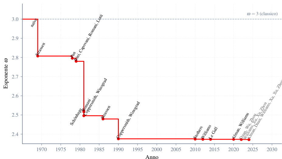
Figura 3.1: Miglioramenti del limite superiore dell'esponente della moltiplicazione matriciale \omega dal 1969 ad oggi. La linea tratteggiata rappresenta il limite superiore \omega < 3 .
