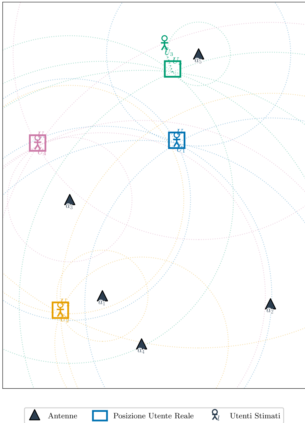
Figura 4.7: Stima della posizione degli utenti e delle antenne in assenza di rumore. I quadrati trasparenti indicano le posizioni reali degli utenti U_r , gli omini indicano le posizioni stimati \hat{U}_r , i triangoli scuri indicano le antenne a_i , e le circonferenze tratteggiate indicano le distanze stimati dalle antenne.
