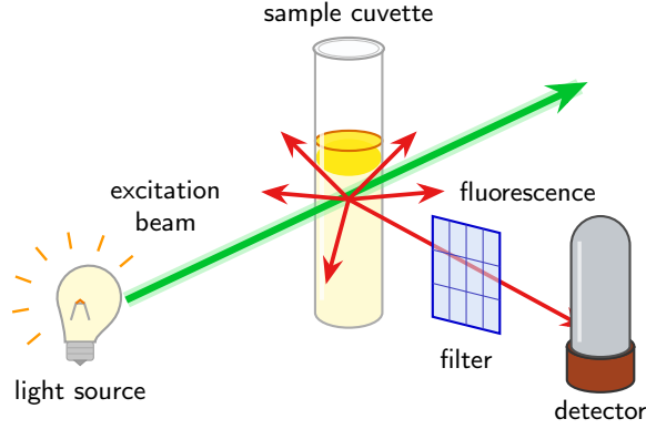
Figura 3.1: Rappresentazione schematica di uno spettrofotometro per spettroscopia di fluorescenza.
