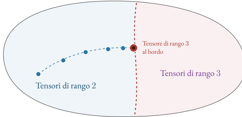
Figura 1.6: Nella varietà dei tensori 2 \times 2 \times 2 una successione di tensori di rango 2 può convergere a un tensore di rango 3 al bordo tra i tensori di rango due e quelli di rango 3.
