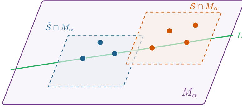
Figura 2.2: Interpretazione geometrica della costruzione nel caso k = 1 ( L è una retta, e gli M_\alpha sono piani). In questo caso L contiene almeno \mu \geq k + 1 = 2 punti di \tilde{\mathcal{S}} , e M_\alpha contiene almeno \mu + 1 \geq k + 2 = 3 di \tilde{\mathcal{S}} ; per ipotesi induttiva, 3 \leq \#(\tilde{\mathcal{S}} \cap M_\alpha) \leq \#(\mathcal{S} \cap M_\alpha) . A priori i punti di \mathcal{S} potrebbero non intersecare L , ma attraverso un conteggio troviamo che 2 \leq \#(\tilde{\mathcal{S}} \cap L) \leq \#(\mathcal{S} \cap L) .
