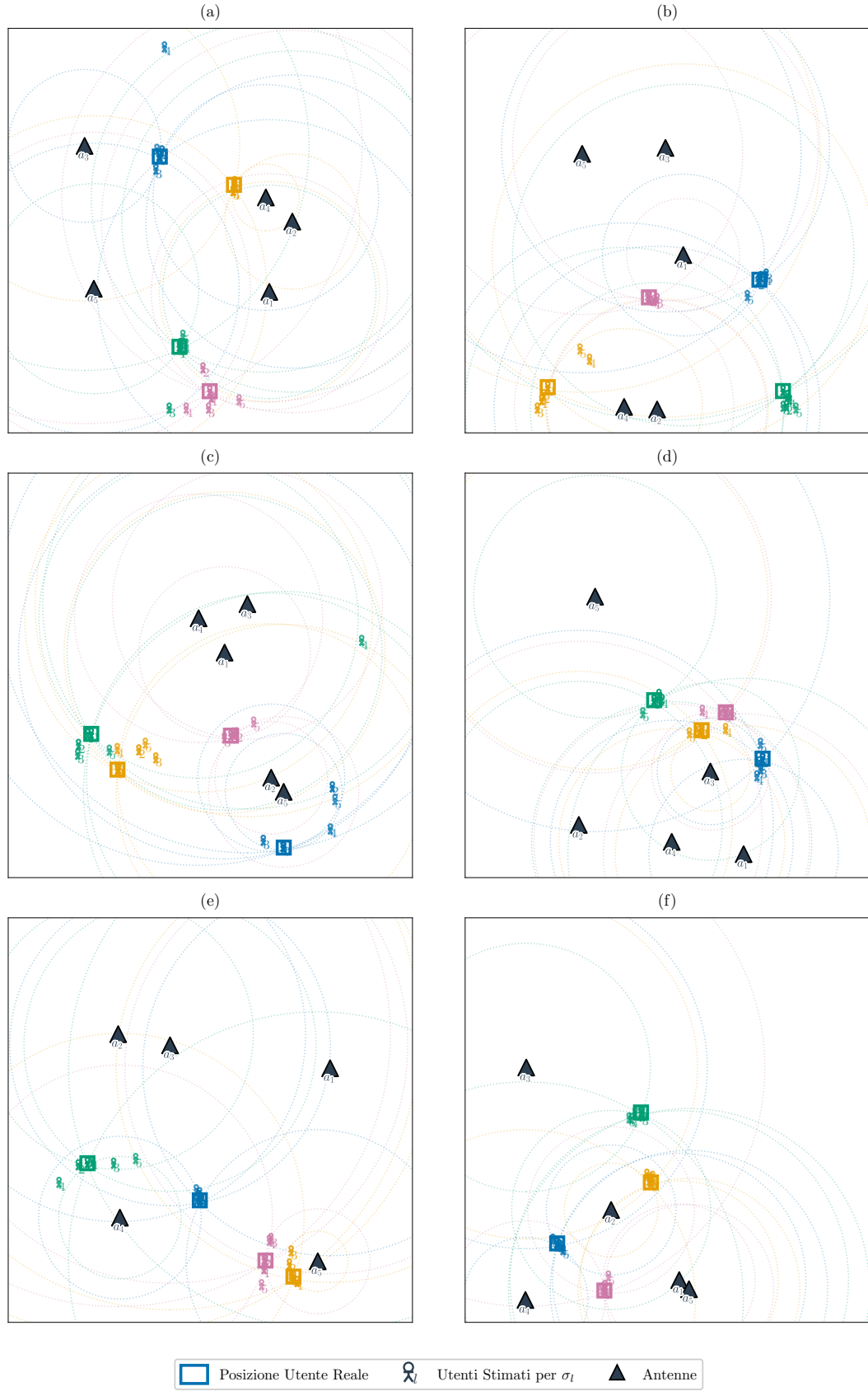
Figura 4.10: Deriva della localizzazione degli utenti sotto rumore gaussiano per sei esperimenti indipendenti (disposizioni spaziali differenti), mostrando i comportamenti tipici di deriva al crescere del livello di rumore \sigma_l .
