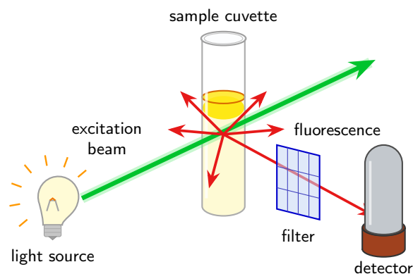
Figura 4.1: Spettrofotometro per spettroscopia di fluorescenza.
