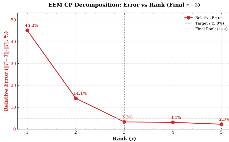
Figura 4.4: Errore relativo al variare del rango della decomposizione approssimante. Il rango ottimale selezionato è r = 3 , corrispondente al superamento della tolleranza target \varepsilon = 0.05 . Osserviamo che la precisione non varia di molto all'aumentare di r .
