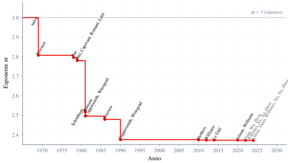
Figura 3.1: Cronologia dei miglioramenti del limite superiore dell'esponente della moltiplicazione matriciale \omega dal 1969 ad oggi. La linea tratteggiata rappresenta il limite superiore banale \omega \leq 3 dato dall'algoritmo classico scolastico.
