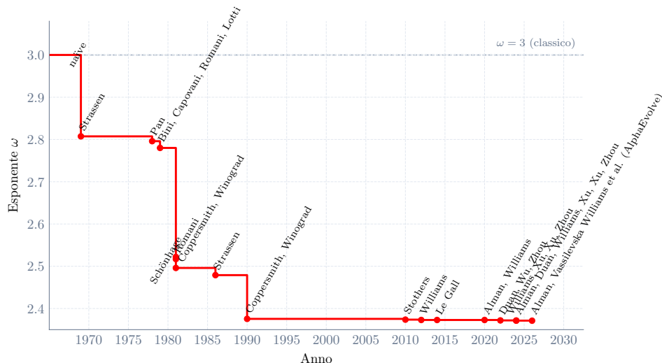
Figura 3.2: Miglioramenti del limite superiore dell'esponente della moltiplicazione matriciale \omega dal 1969 ad oggi. La linea tratteggiata rappresenta il limite superiore \omega < 3 .
