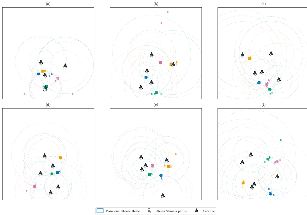
Figura 4.10: Deriva della localizzazione degli utenti sotto rumore gaussiano per sei esperimenti indipendenti (disposizioni spaziali differenti), mostrando i comportamenti tipici di deriva al crescere del livello di rumore \sigma_l .
