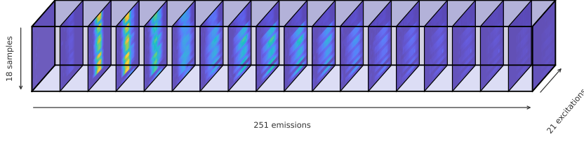
Figura 2.2: Rappresentazione tridimensionale del tensore EEM di dimensioni 18 \times 251 \times 21 .
