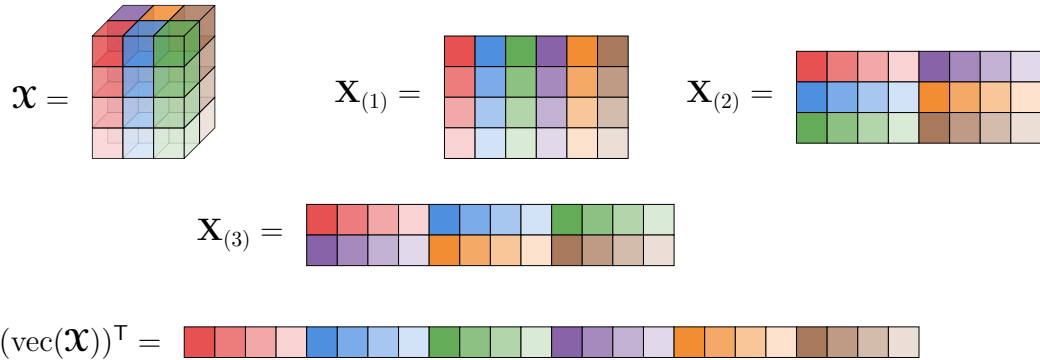
Figura 1.1: Schema delle matricizzazioni di un tensore.
