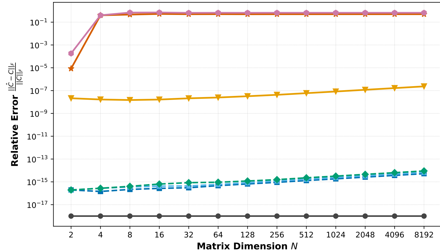
Numerical Relative Error
