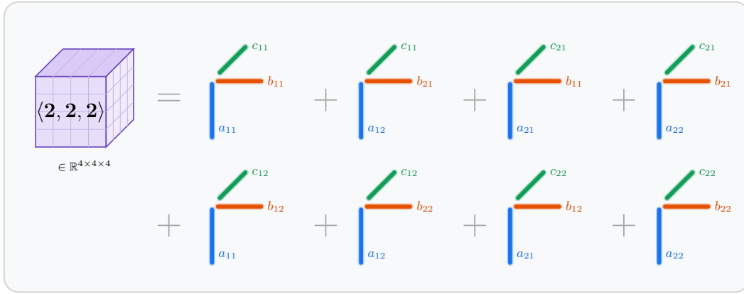
Figura 3.4: Decomposizione CP di rango 8 del tensore di moltiplicazione di matrici \langle 2, 2, 2 \rangle .
