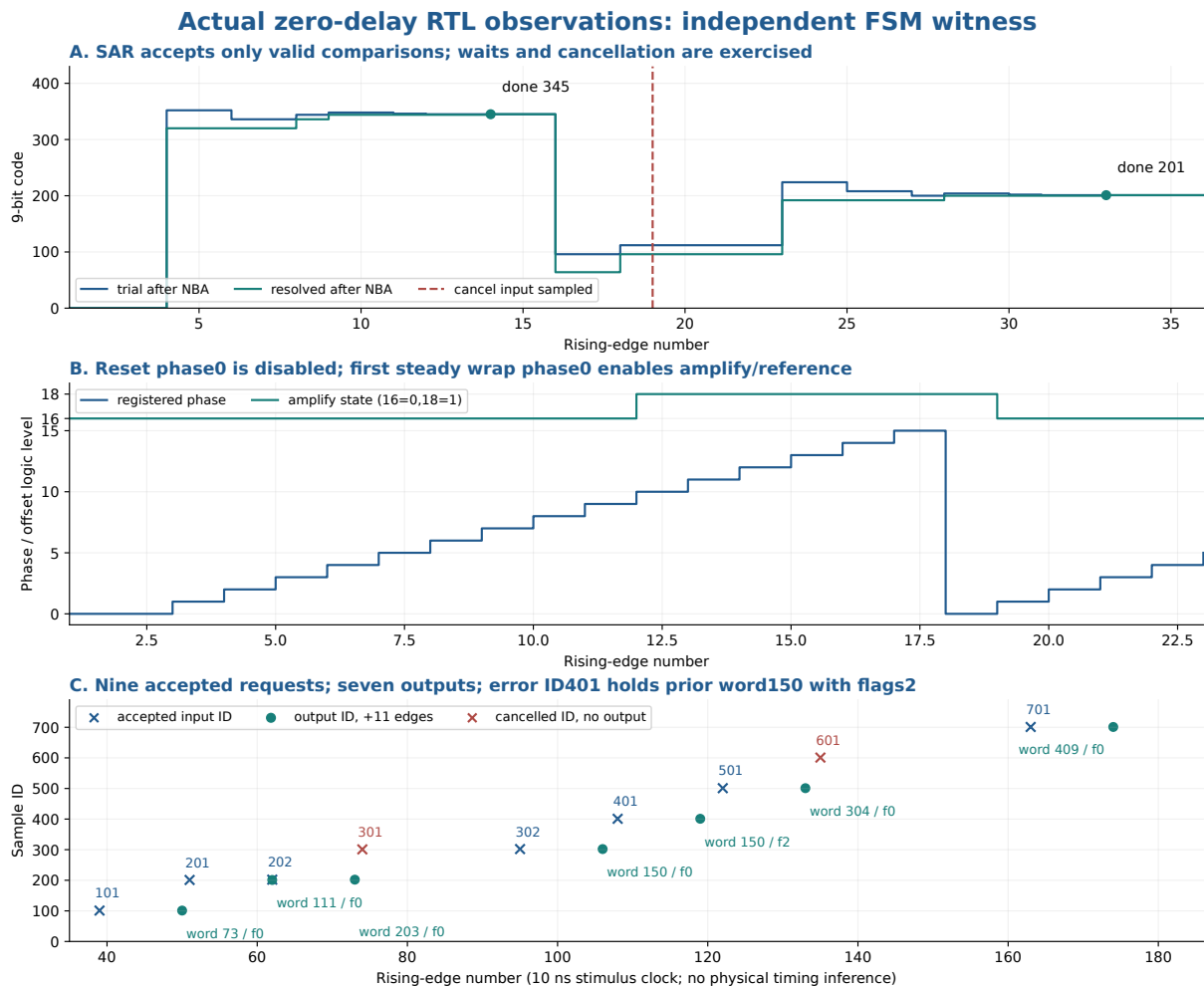
图 12.5: SAR 接受、相位启动与重构完成事件的实际 trace 视图。它与前四幅解释图的角色不同：运行、来源 SHA、信号记录时点及检查范围须同时绑定，不能由状态图插值或补画未观测值。
