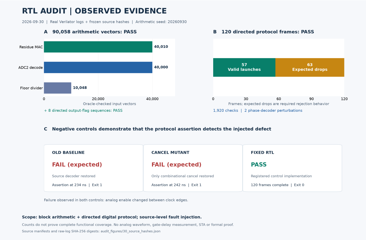
图 7.5: 首轮定向实跑日志与 manifest 的证据概览；后续跨版本审计另立来源。每个计数都有原始数据；图是覆盖样本和判据的展示，不是人为绘制的电路波形。
