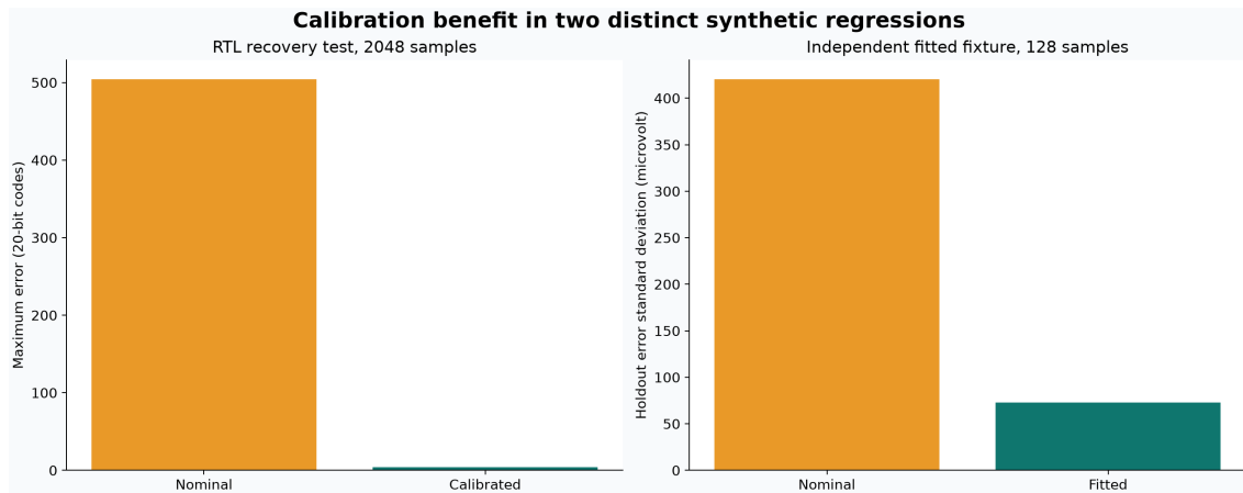
图 7.3: 合成失配的两种校正指标；数值口径不同，不可直接换算为芯片 ENOB。
