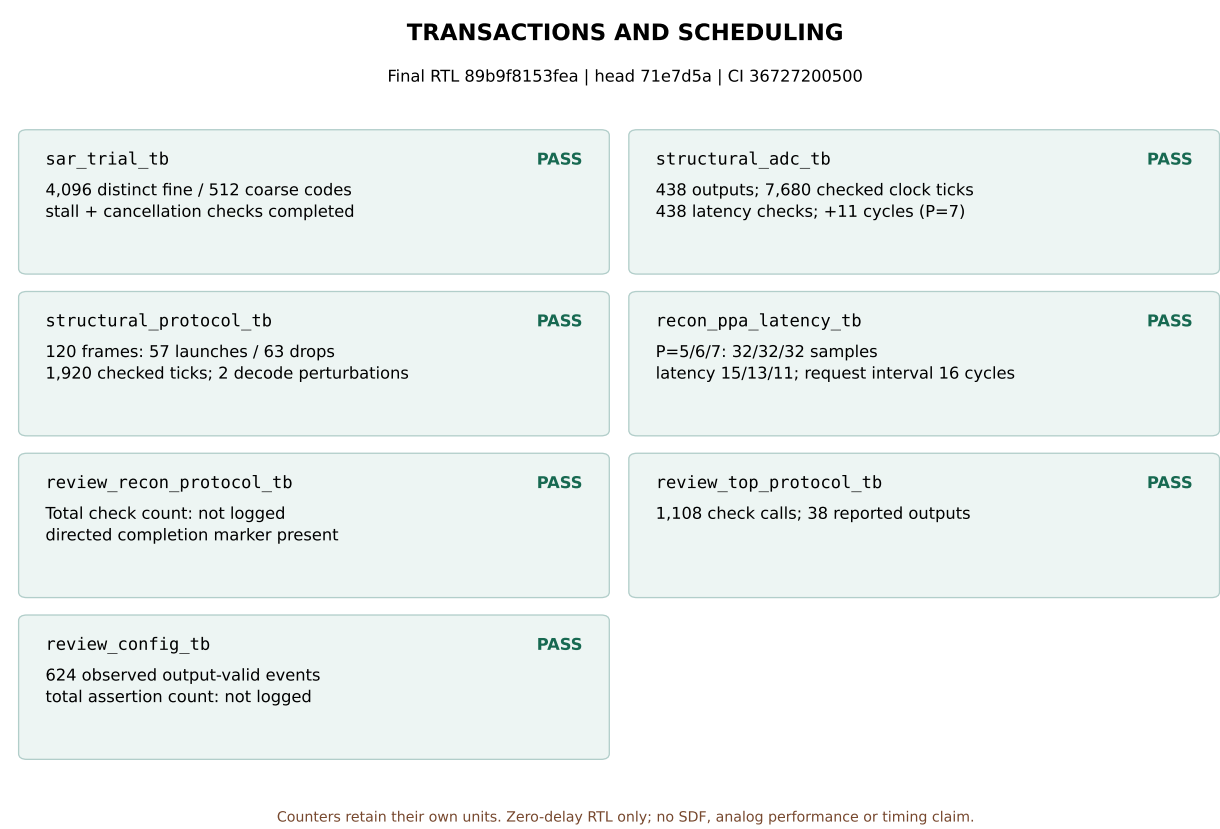
图 11.13: 最终源码七项事务/调度 RTL 证据: 截止取消、上下文与 ID/flags 对齐、配置锁定以及三档连续请求。P5/P6/P7 各 32 笔连续请求间隔 16 拍, 输出延迟 15/13/11 拍; 这是功能拍数, 不是纳秒时序。
