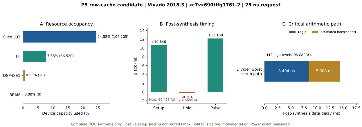
图 11.7: 当前缓存版 P5 的原始 utilization.rpt、timing_summary.rpt 和 timing_paths.rpt 重绘: A 为器件资源占用, B 将 setup/hold/pulse 分开, C 拆出最坏除法路径的逻辑延迟与综合后估算互连延迟。图中 25 ns 为申请约束, hold 负值仍然保留; 脚本与来源哈希见 audit_figures/make_cached_p5_synth_evidence.py 及同名 *.sha256.json。
