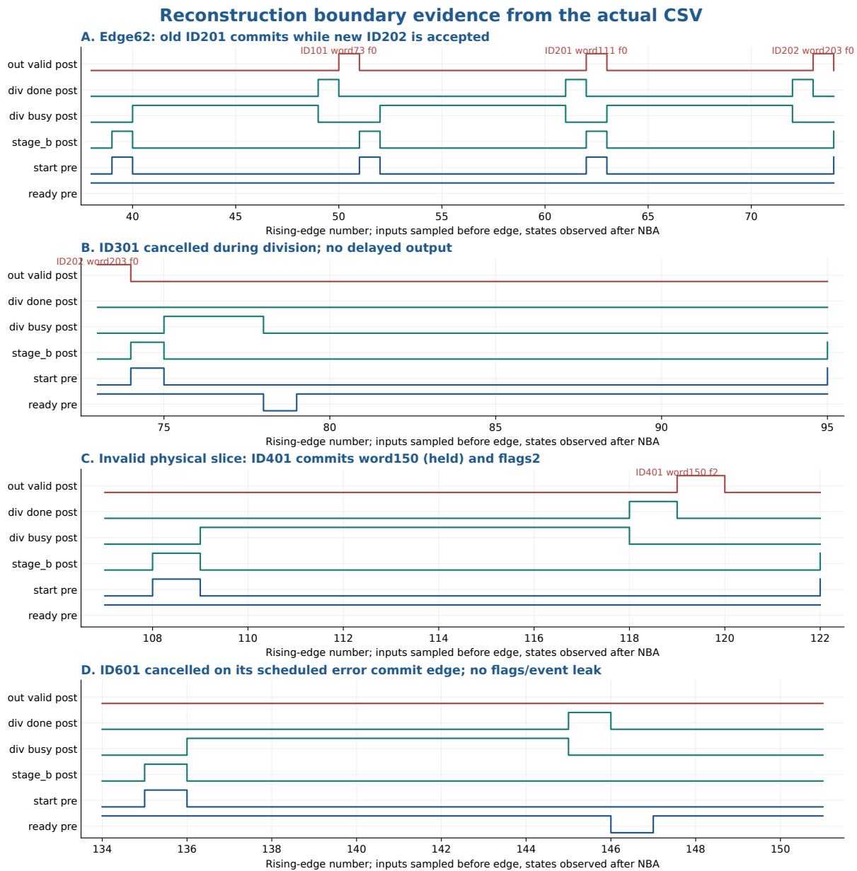
图 12.6: 来自实际重构 CSV 的四段边界记录: 旧结果提交与新 start 同沿、运行中取消、非法 slice 错误提交、错误提交沿取消。输入为沿前值, 状态为 NBA 后值; 不含 SDF 或模拟宏。
