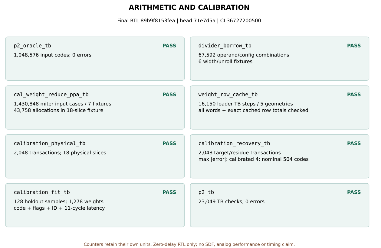
图 11.12: 最终共享读选源码的八项算术/校准 RTL 证据，包含独立行缓存状态检查、四路归约比较、完整码域简化构造、小位宽除法穷举及标定系数应用。每项仍受本身激励与判据范围限制。
