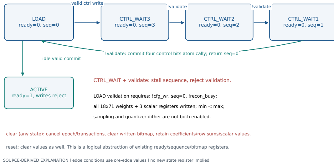
图 12.4: 配置 LOAD、控制等待与 ACTIVE 的逻辑状态解释图。clear 和 reset 效果不同, validate 冲突保持等待序列; 图不是仿真证明, 实际拒写/提交/取消须由配置测试观察。
