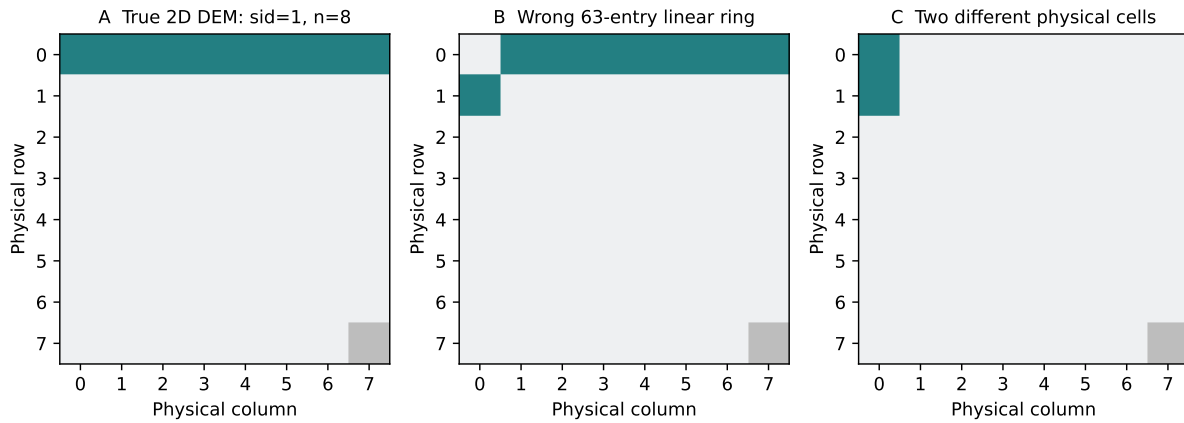
图 11.16: 二维 DEM 不能直接换为一维环的反例: \text{sid}=1 、主计数 8 时, 二维方案选择同一行内循环的八项, 一维方案则跨到下一行, 两项物理单元不同。灰色格为不存在的物理单元 63。这是算法结构与错误候选示意, 非 RTL 仿真波形。
