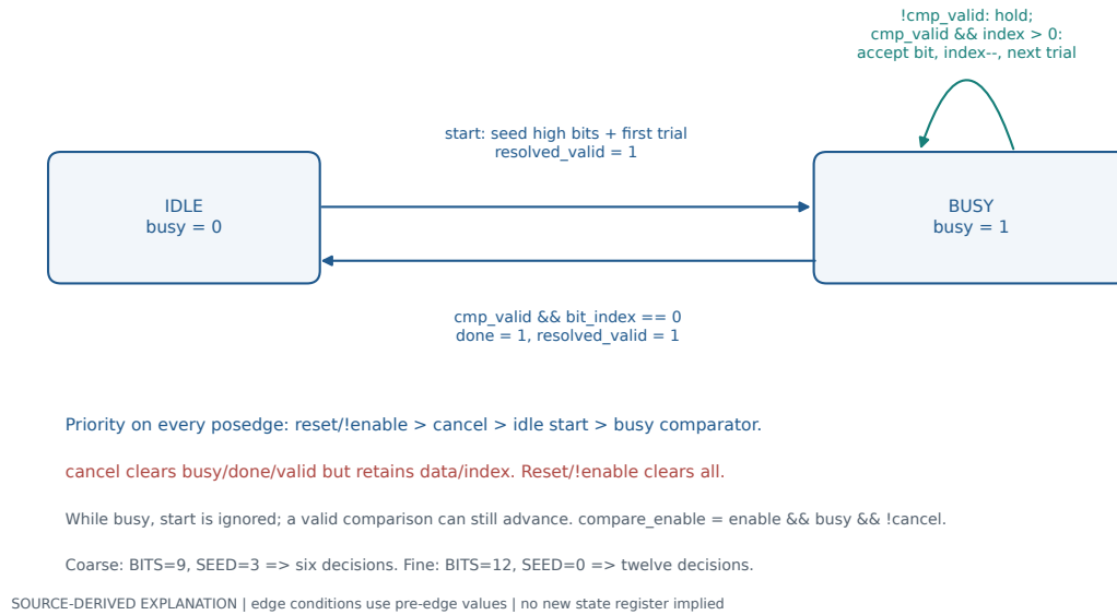
图 12.2: SAR 控制的 IDLE/BUSY 逻辑状态解释图，反映当前 busy/index 编码与转移优先级。它不是仿真证明；转移需由有效比较、停顿、busy start、cancel 与 reset 用例实际覆盖。
