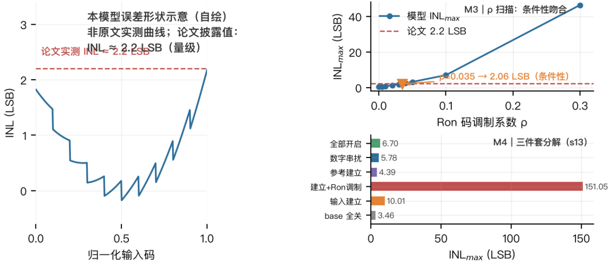
图 4: INL 形态与动态误差机制对照 (M3/M4, [00]) —— 左: 本模型误差形状示意 (自绘, 非原文实测曲线), 论文披露值 \approx 2.2 LSB; 右上: 模型 Ron 码调制扫描 ( s13.ron_sweep ): \rho = 0.035 时 \text{INL}_{\max} = 2.06 \text{ LSB} \approx 论文 2.2 LSB (橙三角标注, 条件性吻合, 取自 s13.rho_max_* ); 右下: 三件套机制对照 ( s13.rows , 单项实验配置与全开不同, 不构成严格可加分解): “输入建立 + Ron 调制” 151 LSB (主导项), 全部开启 6.70 LSB, 参考建立项 4.39 LSB。
