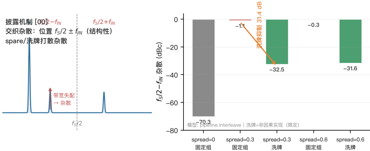
图 3: 交织杂散 (M1/M2, [00]) ——左: 披露机制示意 (自绘): 带宽失配在 f_s/2 \pm f_{IN} 产生结构性杂散, spare/洗牌将其打散; 右: 模型测量 (pipeline.interleave): spread = 0 时该位置为噪声底 -70.3\text{ dBc} , spread = 0.3 固定组 -1.06\text{ dBc} , 洗牌后 -32.46\text{ dBc} ( 31.4 dB , 非因果实现限定, M2)。位置与方向均与披露一致。
