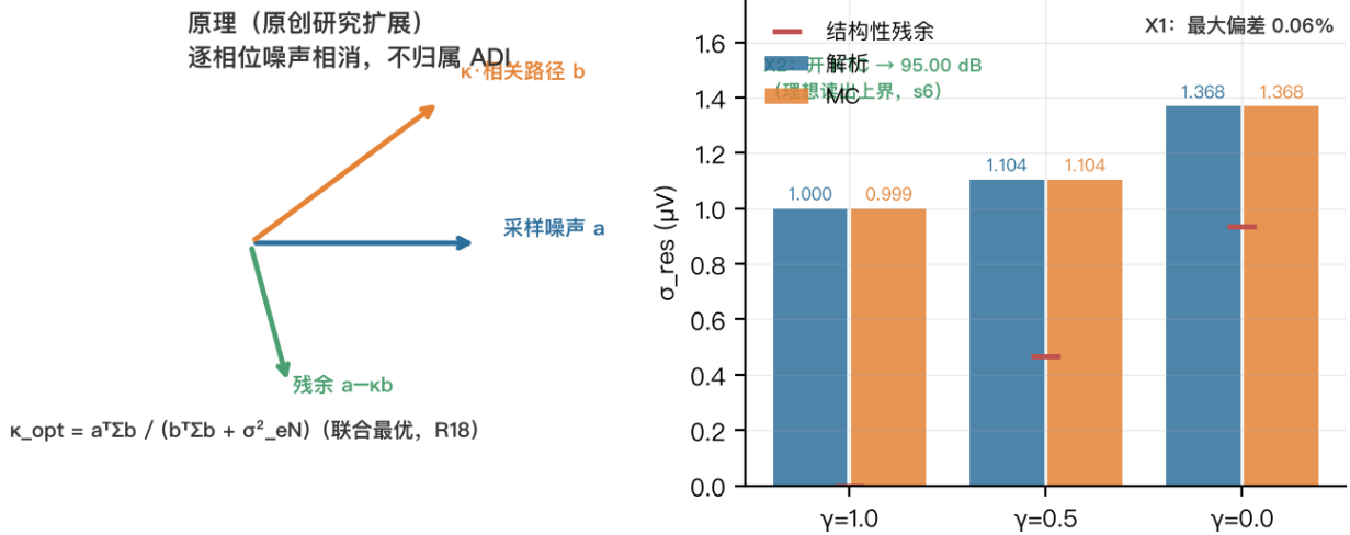
图 8: KTC 逐相位噪声相消 (X1/X2, 原创研究扩展, 不归属 ADI) ——左: 原理示意 (自绘): 采样噪声矢量 a 与相关路径 \kappa b 相消后残余 a - \kappa b , 联合最优 \kappa_{\text{opt}} = a^T \Sigma b / (b^T \Sigma b + \sigma^2_{eN}) (R18 修复); 右: 模型测量 (noise_transfer): \gamma = 1/0.5/0 三覆盖度下 MC (橙) 与解析 (蓝) 的 \sigma_{\text{res}} 对照——最大相对偏差 0.06%, 红色横线为 \gamma < 1 时的结构性残余 ( \gamma = 0 : 0.933 \mu\text{V} )。X2: 开 KTC 后 SNDR 93.70→95.00 dB (理想读出上界)。
