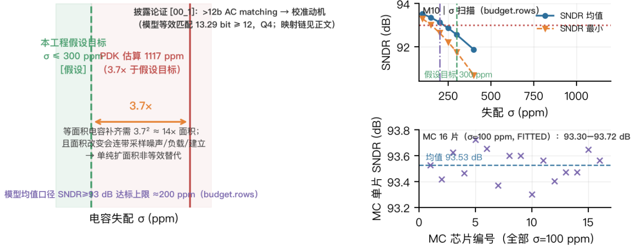
图 7: 失配预算与校准动机 (M10/Q4) ——左: 论证示意 (自绘): 本工程假设目标 300 ppm AS-SUMED vs PDK 估算 1117 ppm (3.7×), 等面积补偿需 \approx 14\times 电容且连带采样噪声/负载/建立——校准是更可行路径; 右: 模型测量 (budget.rows): \sigma 扫描的 SNDR 均值/最小值曲线与 93 dB 目标线; 紫点线为模型均值口径达标上限 \approx 200 \text{ ppm} (与假设目标 300 ppm 是两个口径); 下: MC 16 片 (横轴为芯片编号, 全部芯片同一 \sigma = 100 \text{ ppm} 配置) ( \sigma = 100 \text{ ppm} 配置组, 横轴即该组失配), 分布 93.30–93.72 dB。
