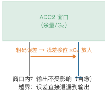
披露机制 [09] §1.3 量化器分离 + 误差自愈窗口
