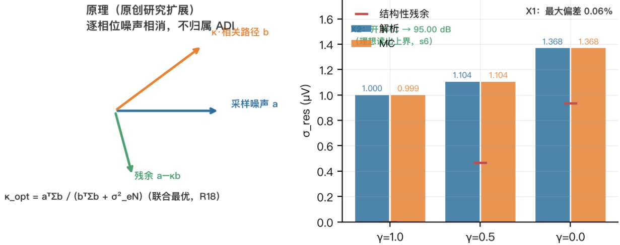
图 8: KTC 逐相位噪声相消 (X1/X2, 原创研究扩展, 不归属 ADI) ——左: 原理示意 (自绘): 采样噪声矢量 a 与相关路径 \kappa b 相消后残余 a - \kappa b , 联合最优 \kappa_{\text{opt}} = a^T \Sigma b / (b^T \Sigma b + \sigma_{eN}^2) (R18 修复); 右: 模型测量 (noise_transfer): \gamma = 1/0.5/0 三覆盖度下 MC (橙) 与解析 (蓝) 的 \sigma_{\text{res}} 对照——最大相对偏差 0.06% , 红色横线为 \gamma < 1 时的结构性残余 ( \gamma = 0 : 0.933 \mu\text{V} )。X2: 开 KTC 后 SNDR 93.70→95.00 dB (理想读出上界)。
