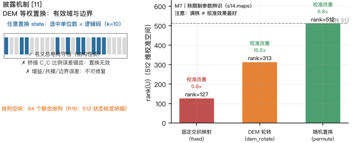
图 5: DEM 有效域与可观测性 (M5/M6/M7, [11]) ——左: 披露机制示意 (自绘): 等权置换保名义守恒, 但 C_C 锯齿/增益/共模/边界误差不在修复域, 联合排列空间为 64 (R16, 排列空间与矩阵秩是两个不同对象); 右: 模型测量 (s14.maps、s14.calibration): 三种映射的 rank(U) (127/313/512) 与整数码校准改善倍数 ( 0.8\times/15.5\times/6.8\times ) ——秩限制参数辨识, 但满秩 \neq 校准效果最好。
