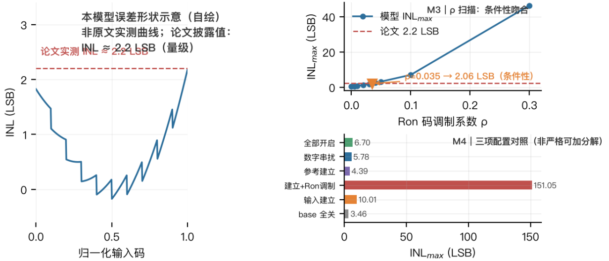
图 4: INL 形态与动态误差机制对照 (M3/M4, [00]) —— 左: 本模型误差形状示意 (自绘, 非原文实测曲线), 论文披露值 \approx 2.2 LSB; 右上: 模型 Ron 码调制扫描 ( s13.ron_sweep ): \rho = 0.035 时 INL_{max} = 2.06 LSB \approx 论文 2.2 LSB (橙三角标注, 条件性吻合, 取自 s13.rho_max_* ); 右下: 三件套机制对照 ( s13.rows , 单项实验配置与全开不同, 不构成严格可加分解): “输入建立 + Ron 调制”151 LSB (主导项), 全部开启 6.70 LSB, 参考建立项 4.39 LSB。
