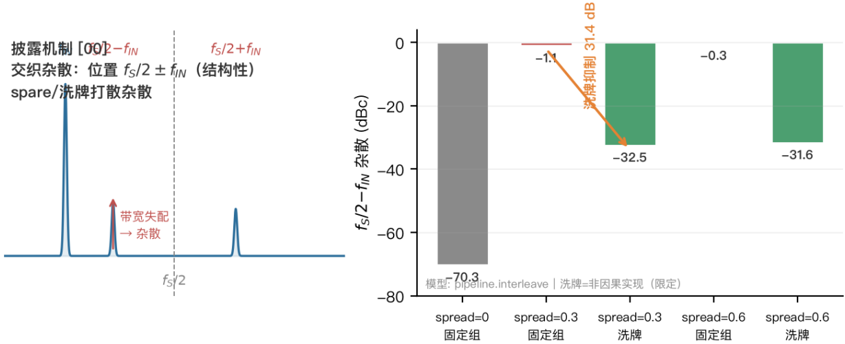
图 3: 交织杂散 (M1/M2, [00]) ——左: 披露机制示意 (自绘): 带宽失配在 f_s/2 \pm f_{IN} 产生结构性杂散, spare/洗牌将其打散; 右: 模型测量 (pipeline.interleave): spread = 0 时该位置为噪声底 -70.3 dBc, spread = 0.3 固定组 -1.06 dBc, 洗牌后 -32.46 dBc (31.4 dB, 非因果实现限定, M2)。位置与方向均与披露一致。
