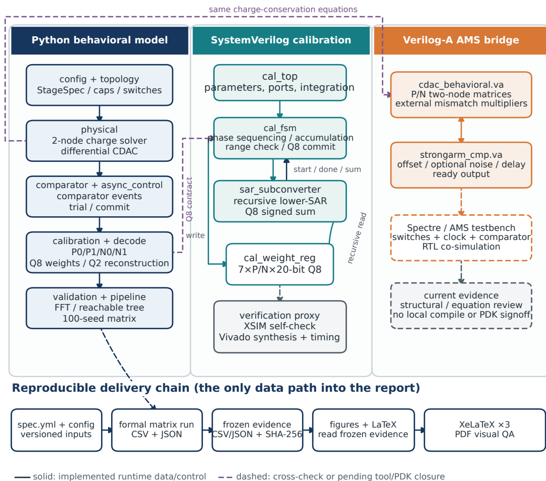
图 1: 工程总架构与证据流。图内统一使用英文。实线是当前实现中的运行时数据/控制；虚线是跨语言等价格检查或尚待工具/PDK 闭环的接口。
