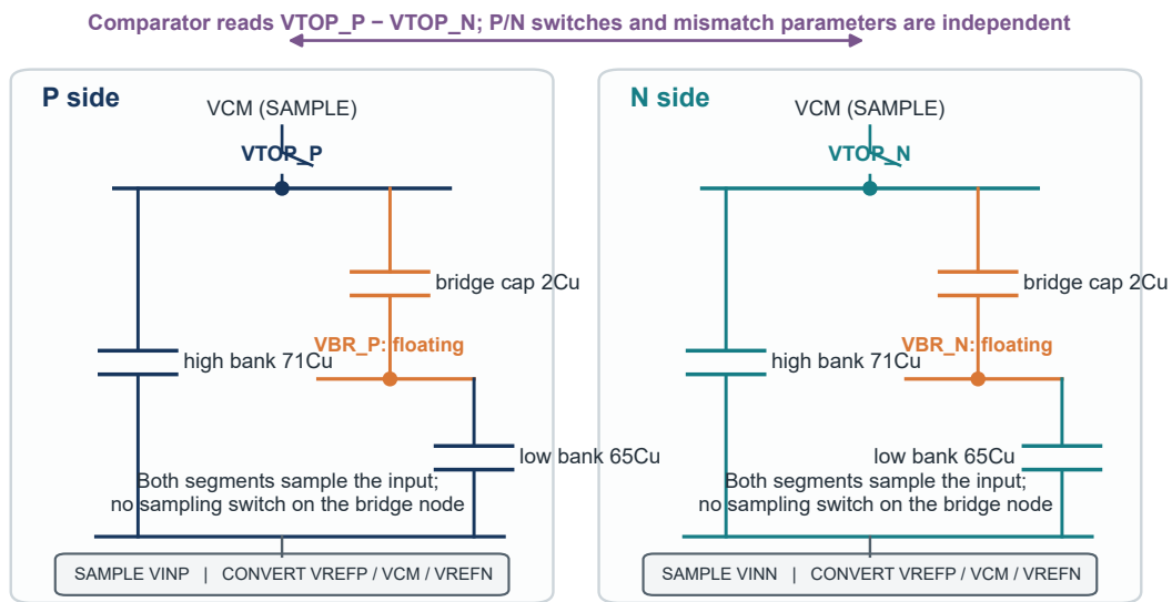
图 2: P/N 两侧完整连接。sampling 只钳位 top node 到 VCM；high/low bottom plates 全部接 VINP/VINN；bridge node 保持浮动。
