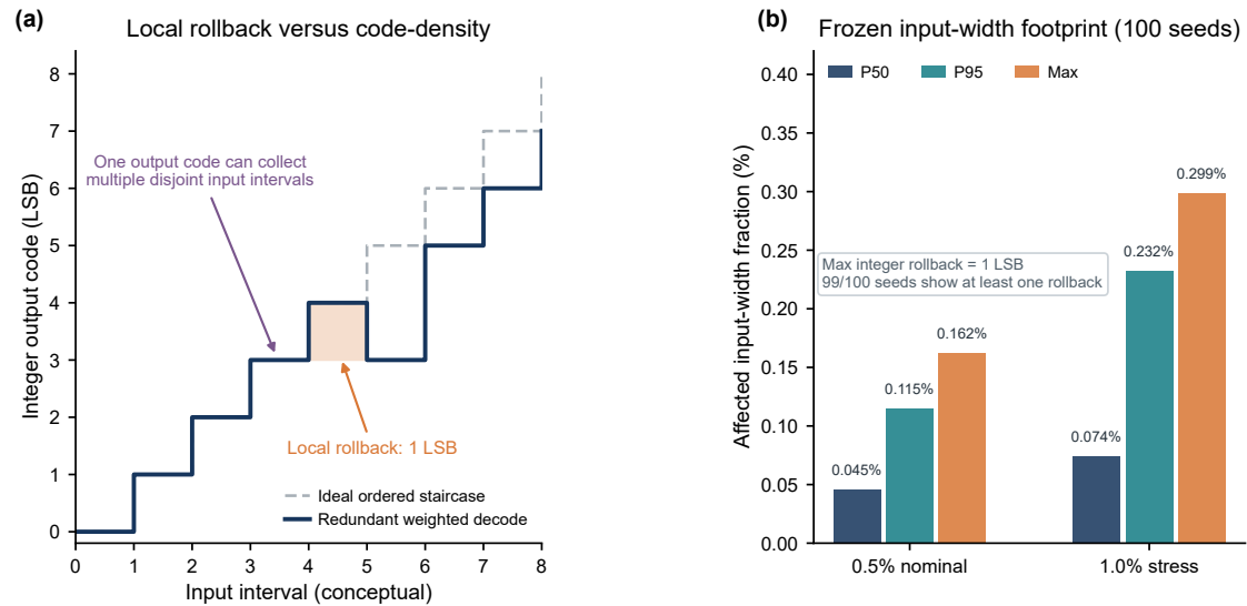
图 6: 左: 局部 1-LSB 回退与 code-density 合并区间的概念示意; 右: 正式 nominal/stress 的受影响输入宽度。
