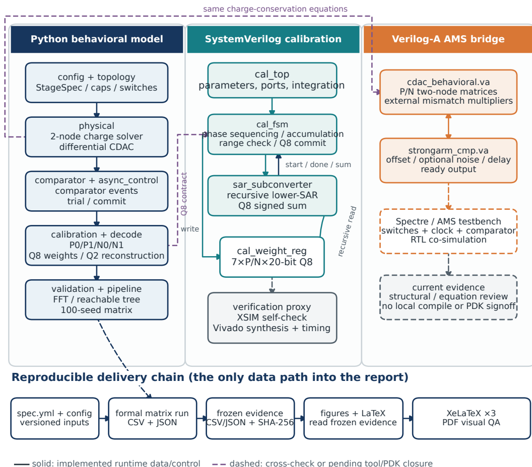
图 1: 工程总架构与证据流。图内统一使用英文。实线是当前实现中的运行时数据/控制；虚线是跨语言等价检查或尚待工具/PDK 闭环的接口。
