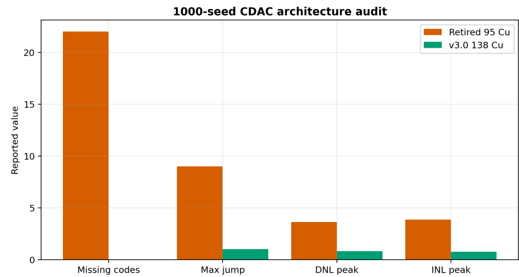
图 14: 旧 95-Cu vs 新 138-Cu CDAC 拓扑对比
