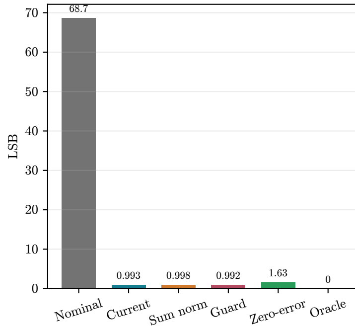
INL max median
