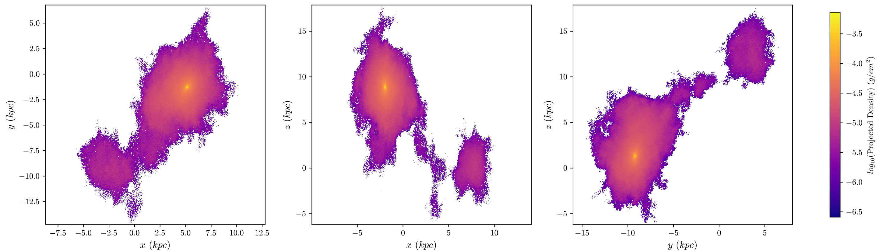
halo8 Dark Matter, z = 3.822 , 512 bins
