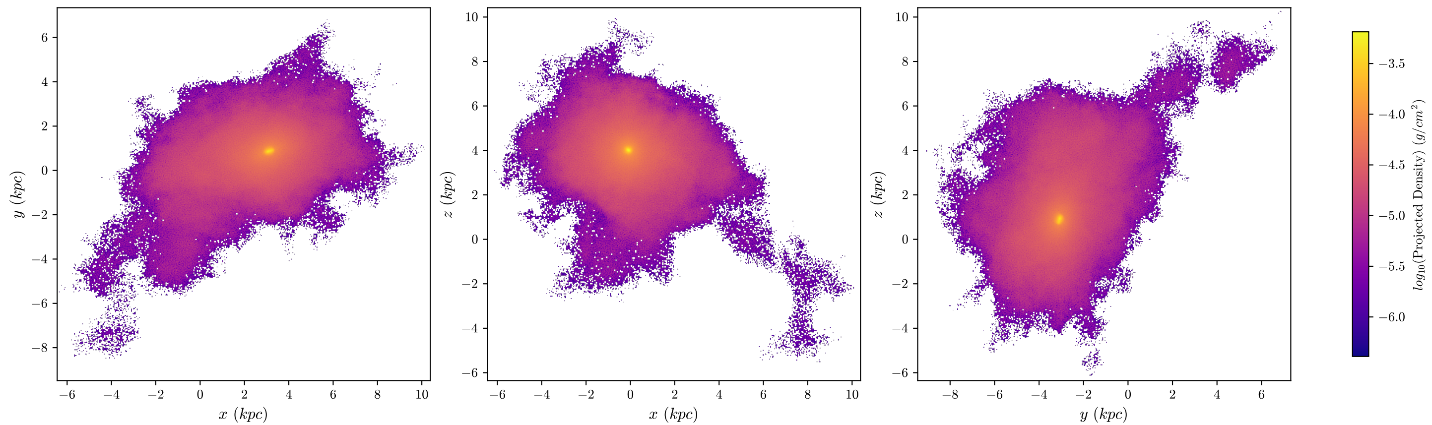
halo8 Dark Matter, z = 3.776 , 512 bins
