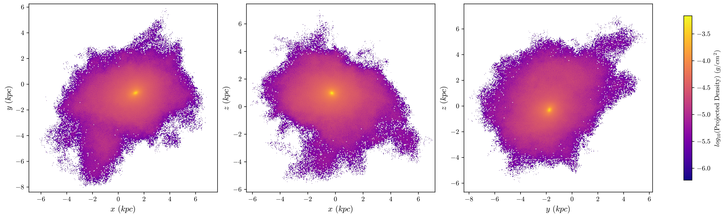
halo8 Dark Matter, z = 3.687 , 512 bins
