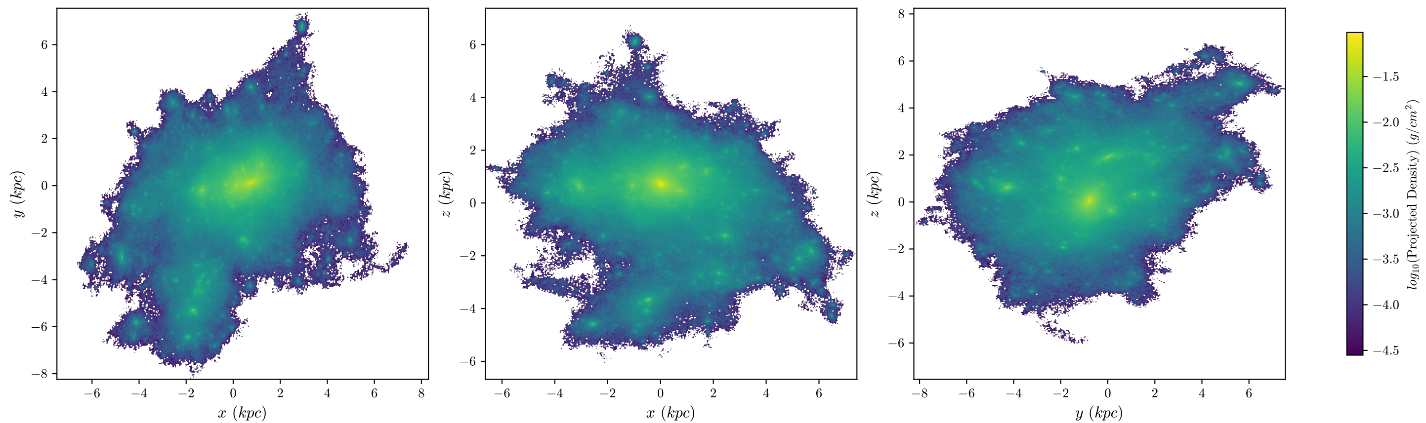
halo8 Stars, z = 3.642 , 512 bins
