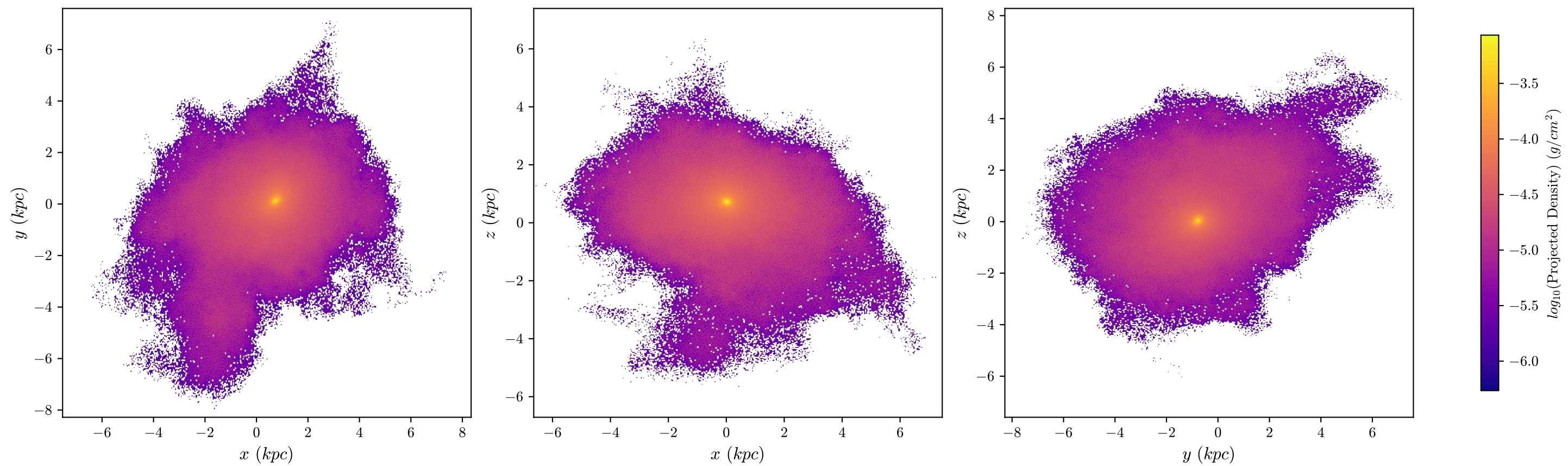
halo8 Dark Matter, z = 3.642 , 512 bins
