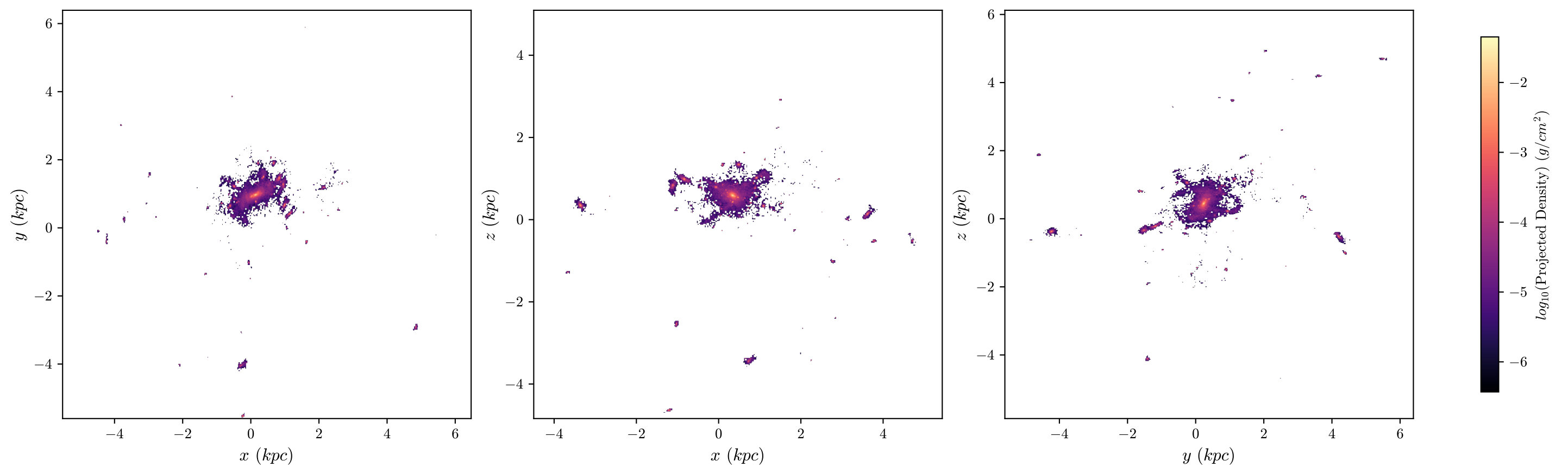
halo8 Stars, z = 3.491 , 512 bins
