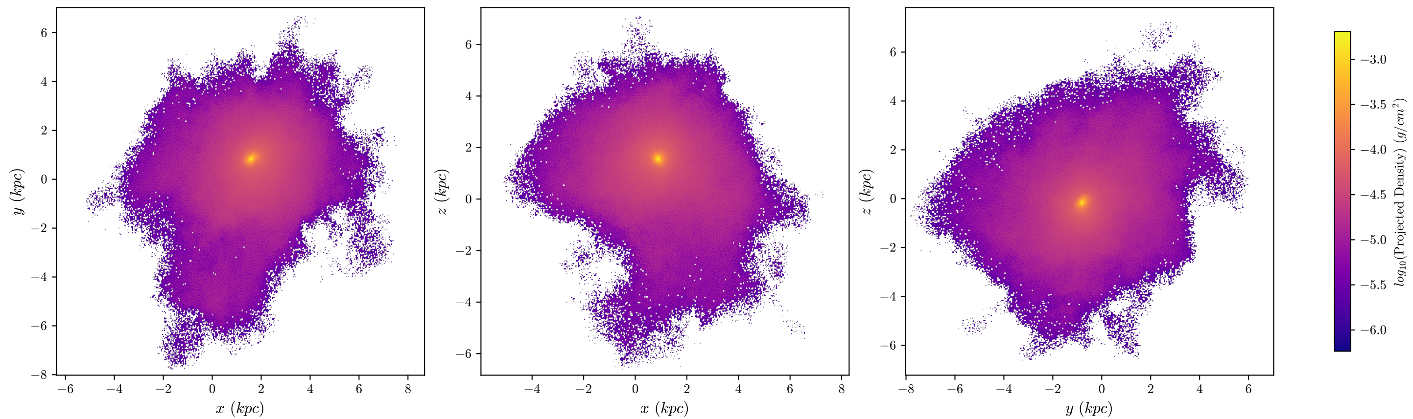
halo8 Dark Matter, z = 3.491 , 512 bins
