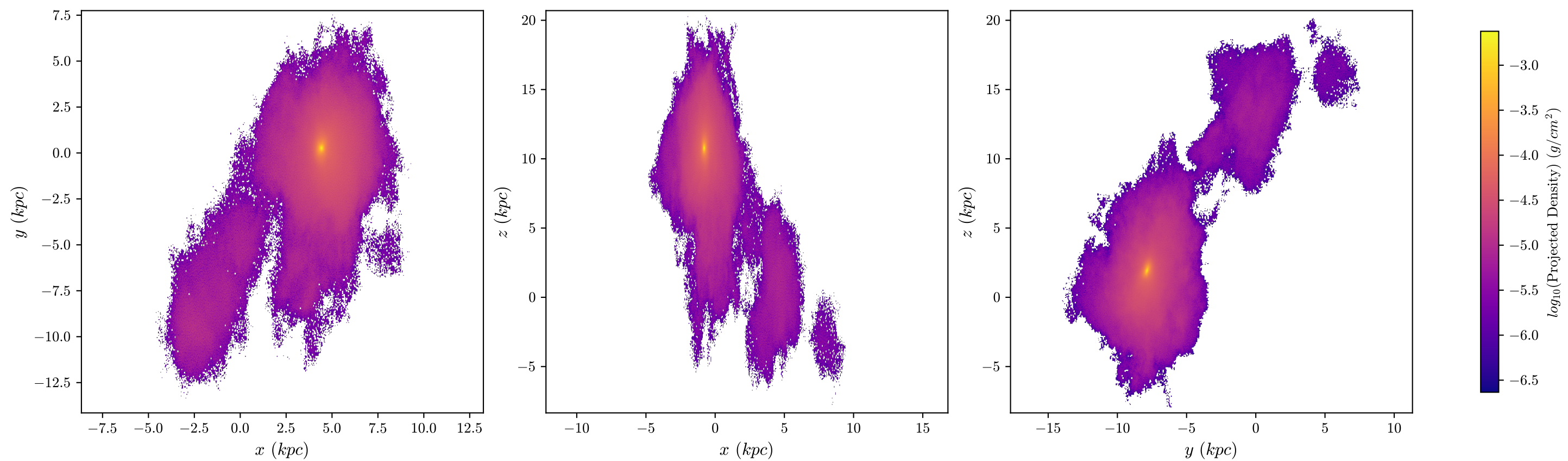
halo8 Dark Matter, z = 3.365 , 512 bins
