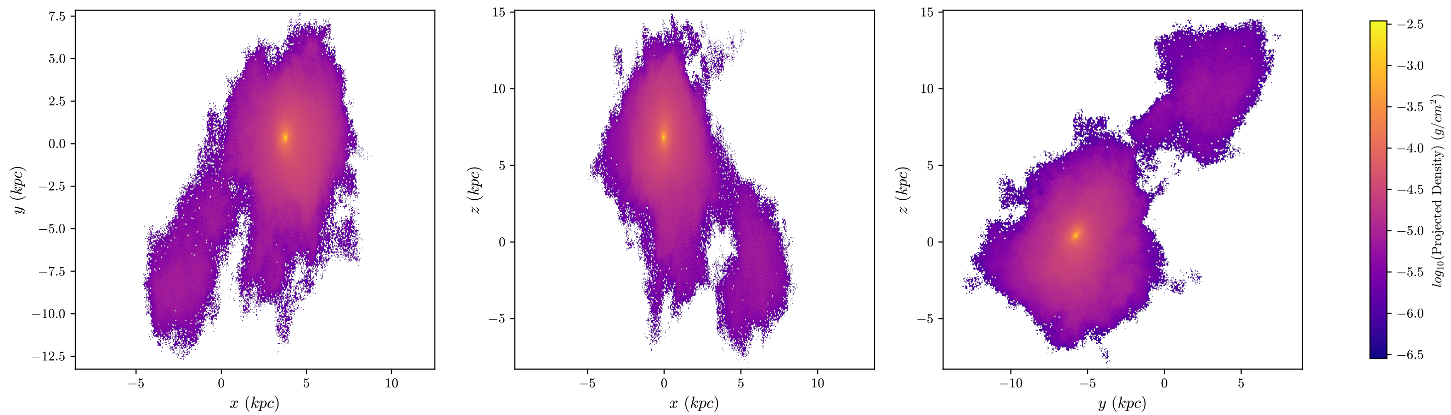
halo8 Dark Matter, z = 3.324 , 512 bins
