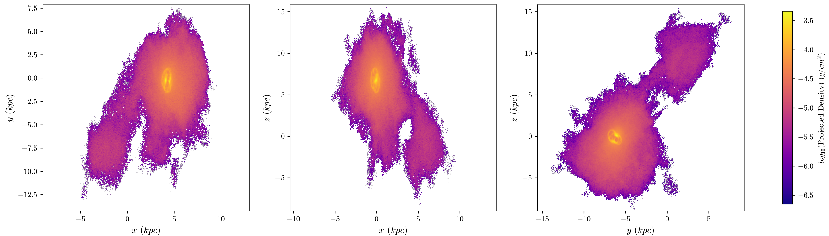
halo8 Dark Matter, z = 3.263 , 512 bins
