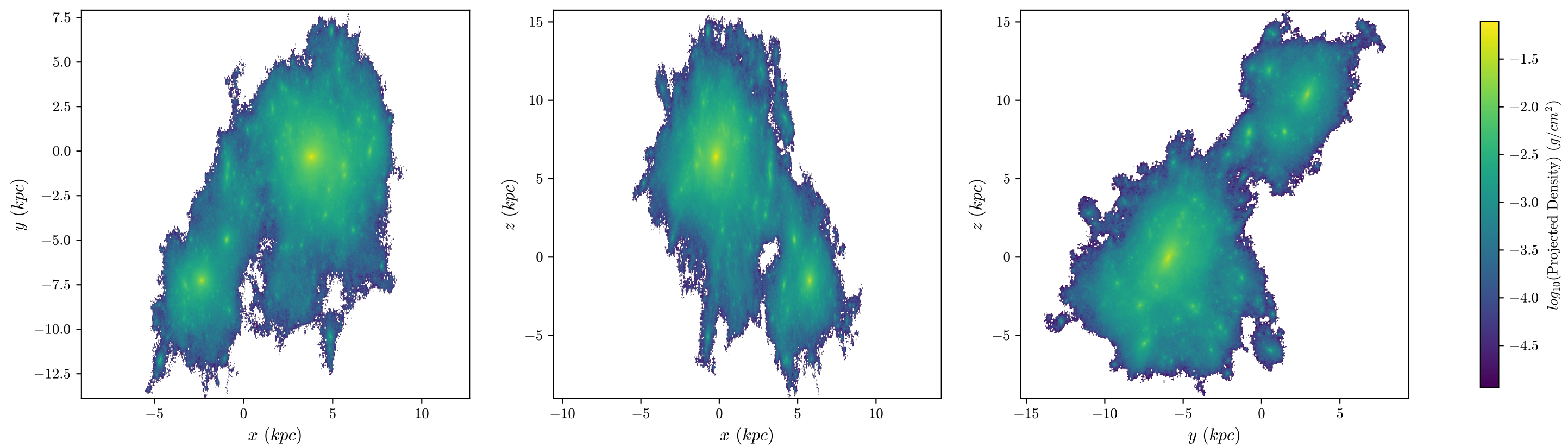
halo8 Dark Matter, z = 3.243 , 512 bins
