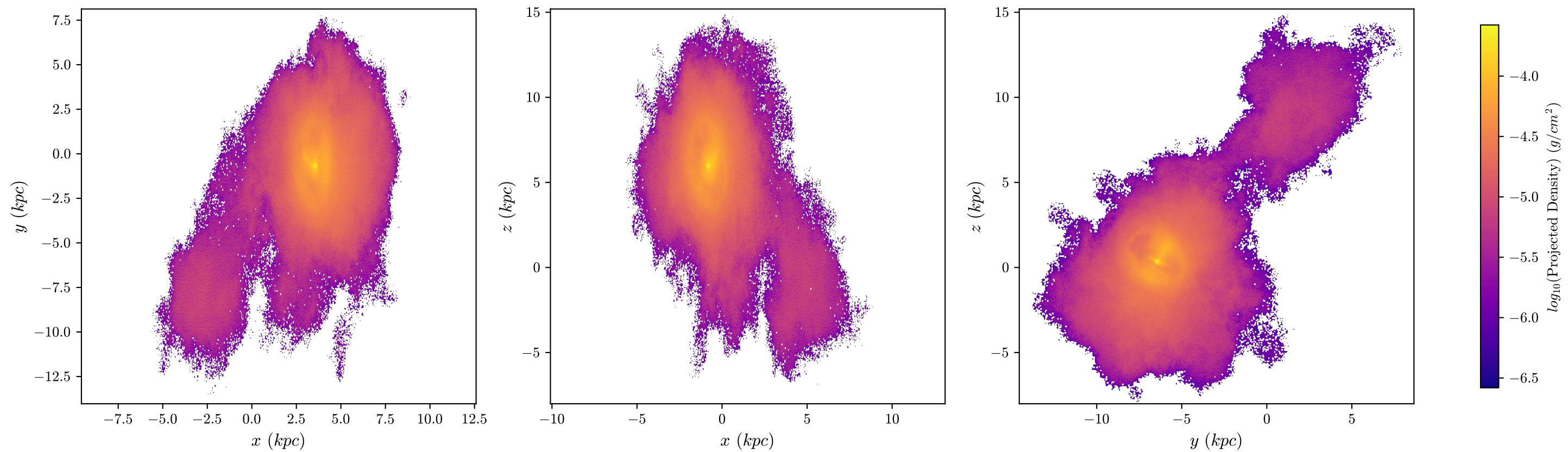
halo8 Dark Matter, z = 3.203 , 512 bins
