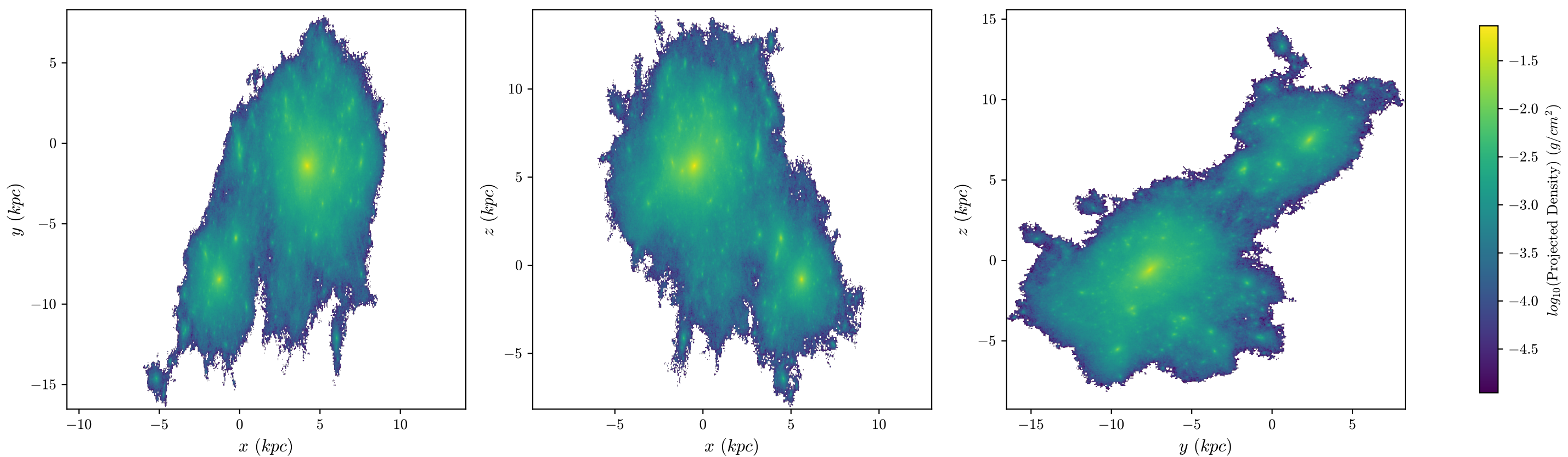
halo8 Stars, z = 3.163 , 512 bins
