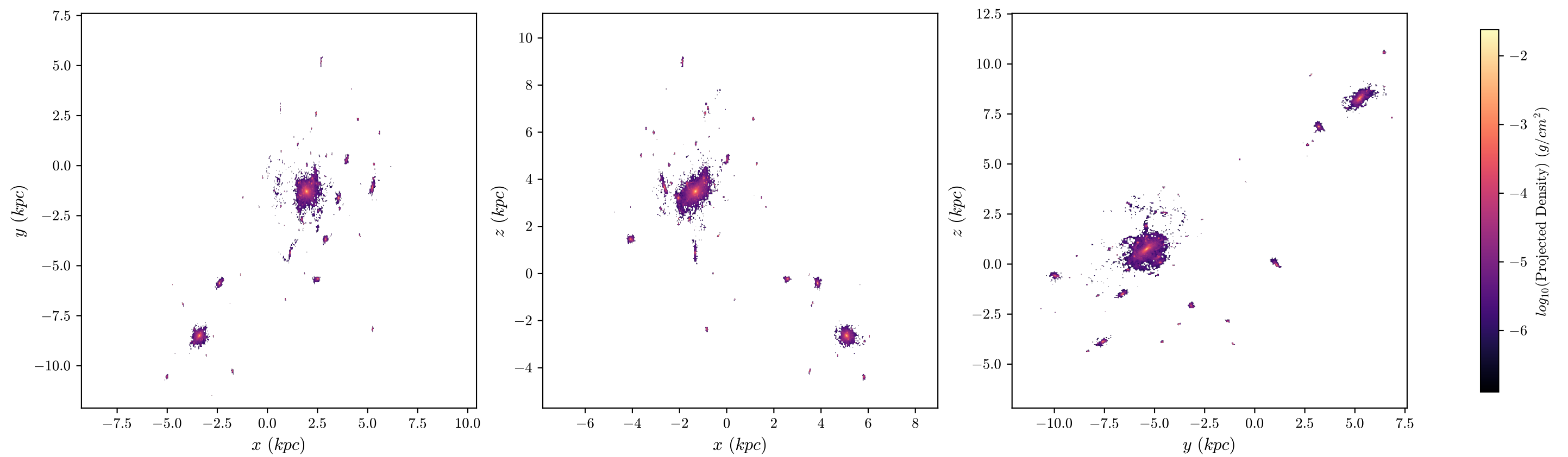
halo8 Stars, z = 3.163 , 512 bins
