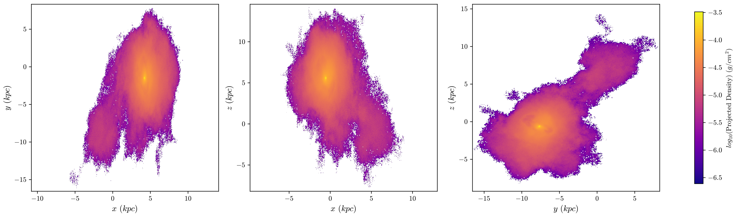
halo8 Dark Matter, z = 3.163 , 512 bins
