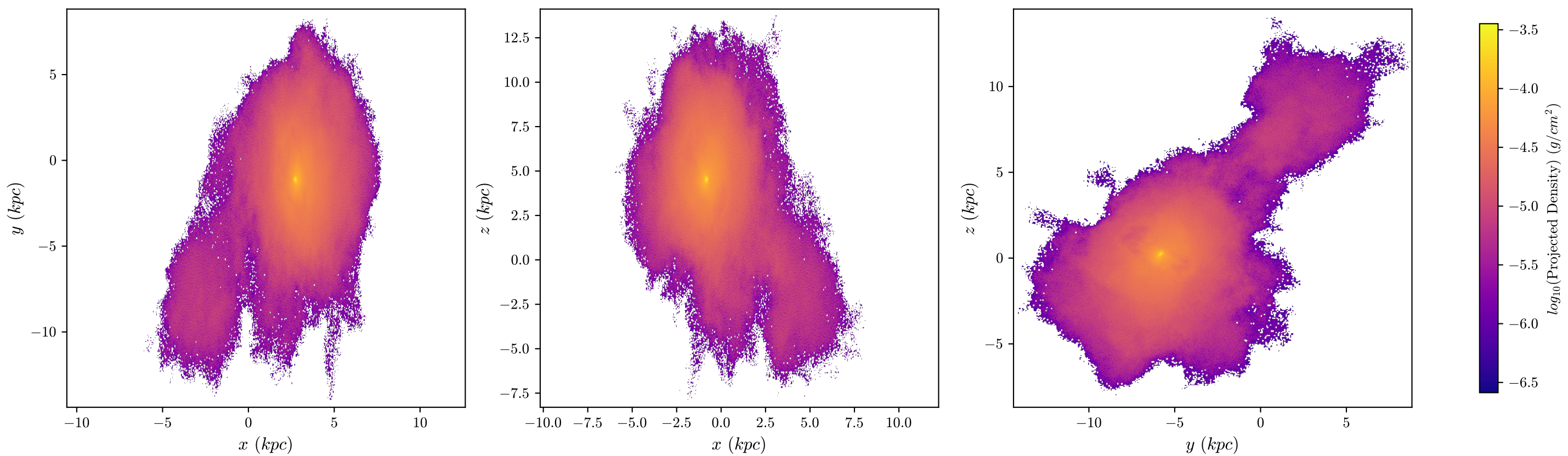
halo8 Dark Matter, z = 3.143 , 512 bins
