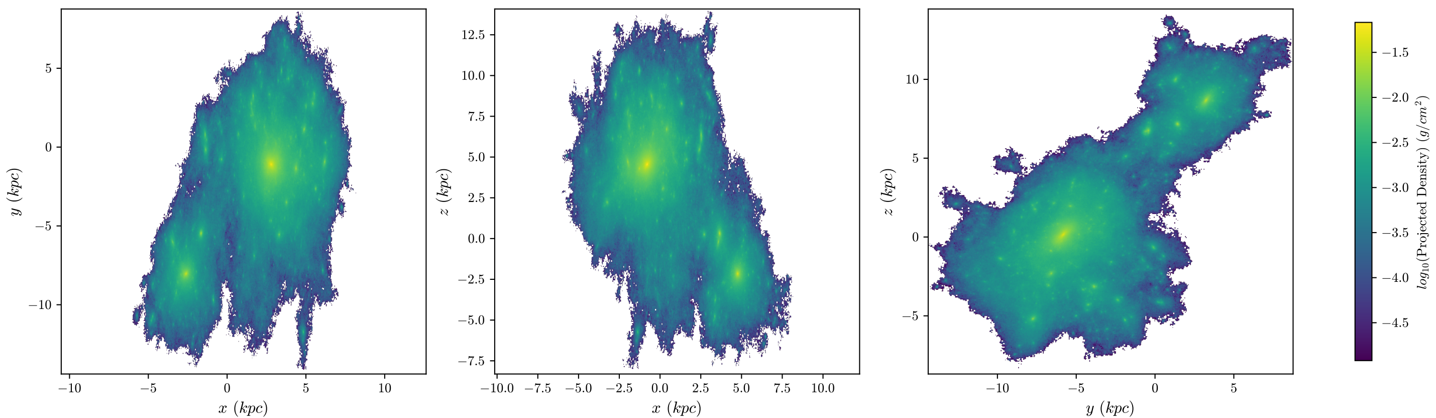
halo8 Stars, z = 3.143 , 512 bins
