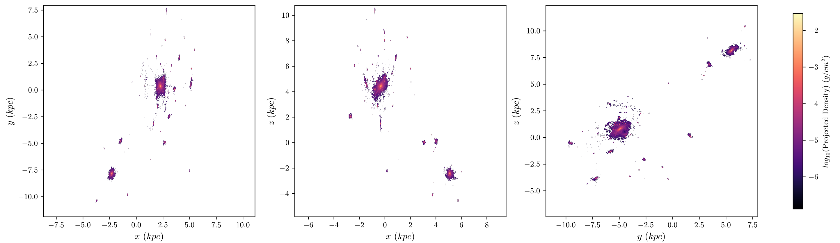
halo8 Stars, z = 3.143 , 512 bins
