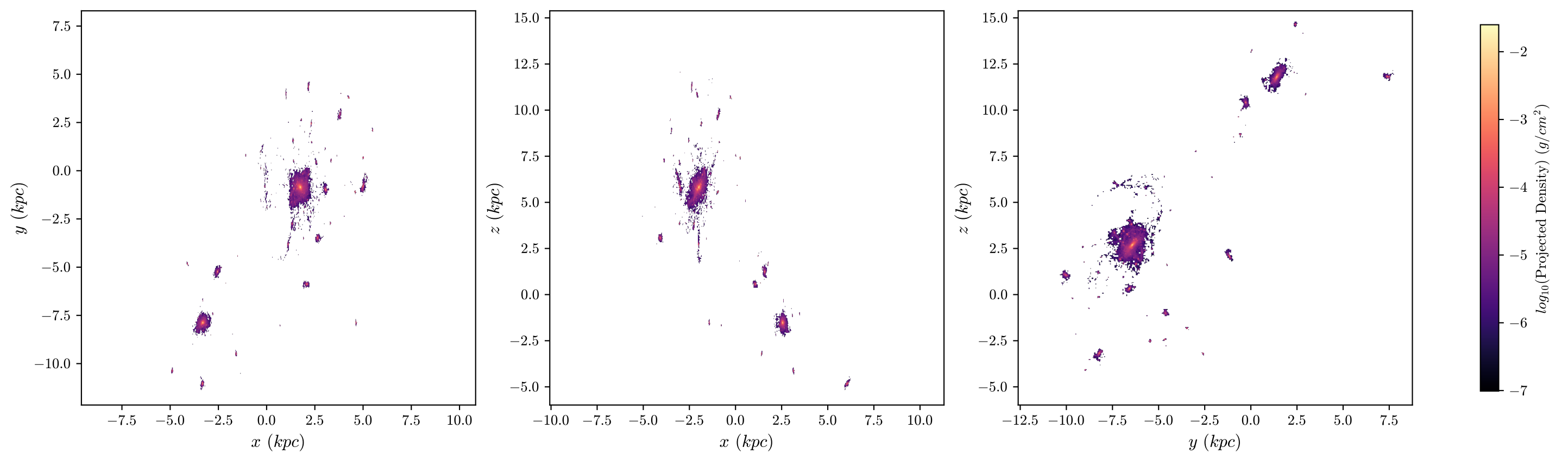
halo8 Stars, z = 3.104 , 512 bins
