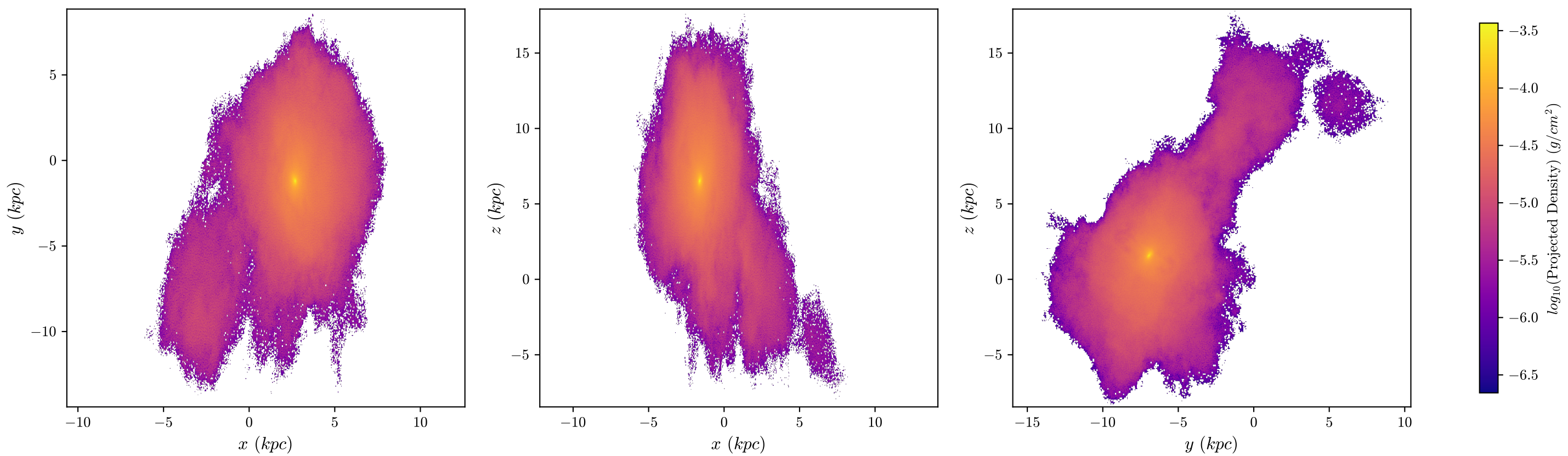
halo8 Dark Matter, z = 3.104 , 512 bins
