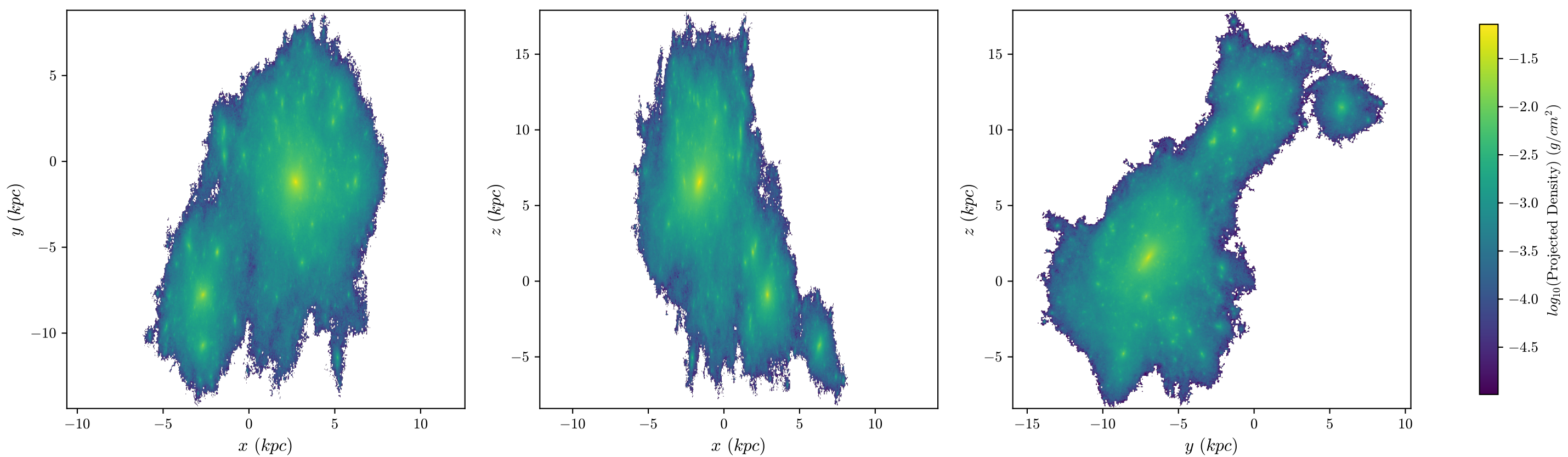
halo8 Stars, z = 3.104 , 512 bins
