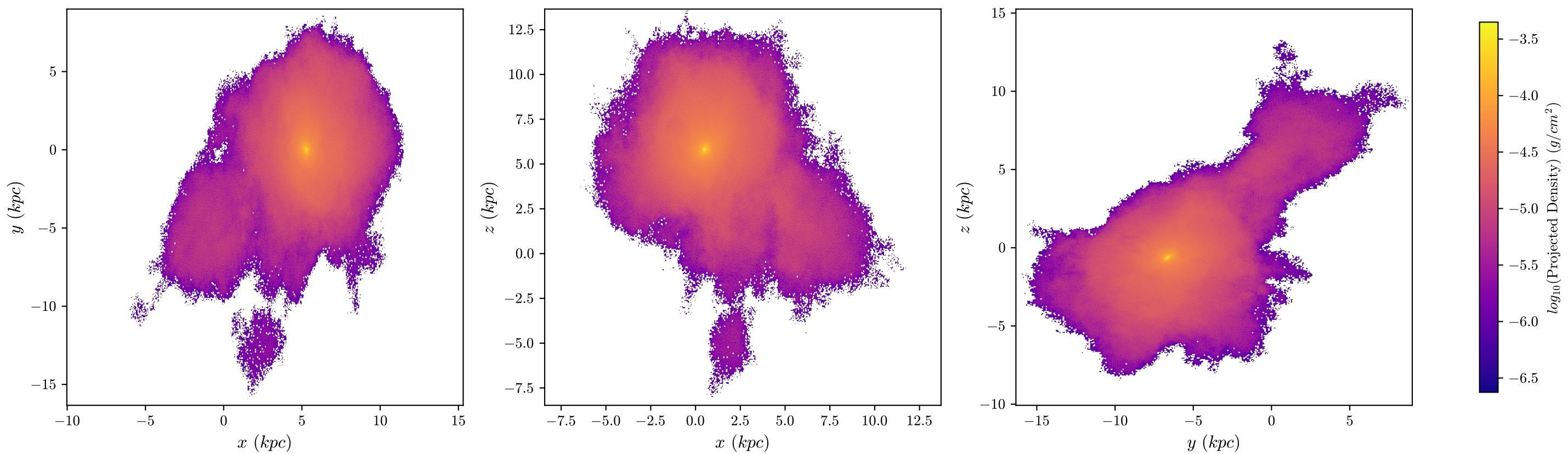
halo8 Dark Matter, z = 3.085 , 512 bins
