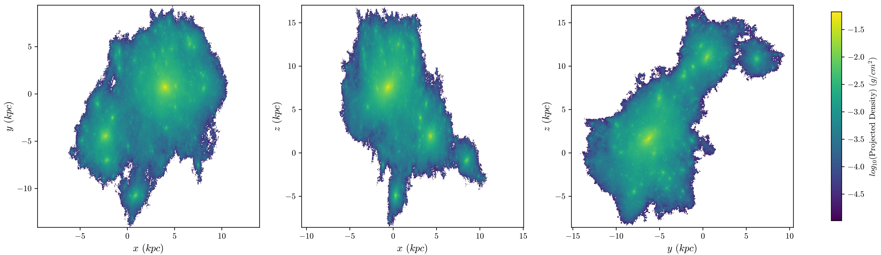
halo8 Stars, z = 3.046 , 512 bins
