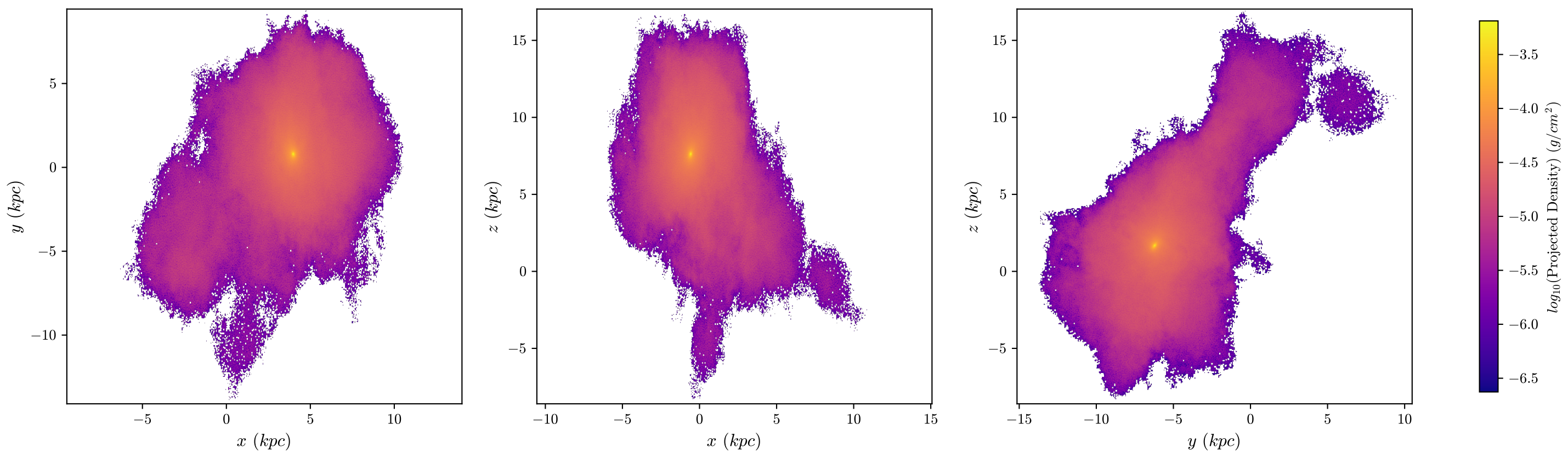
halo8 Dark Matter, z = 3.046 , 512 bins
