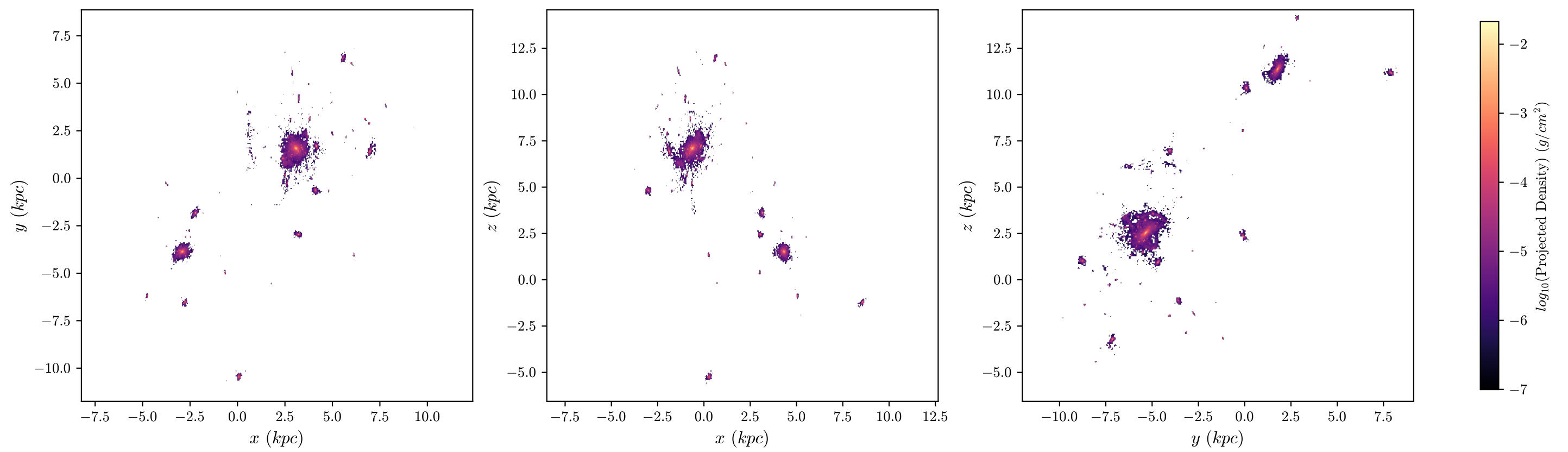
halo8 Stars, z = 3.046 , 512 bins
