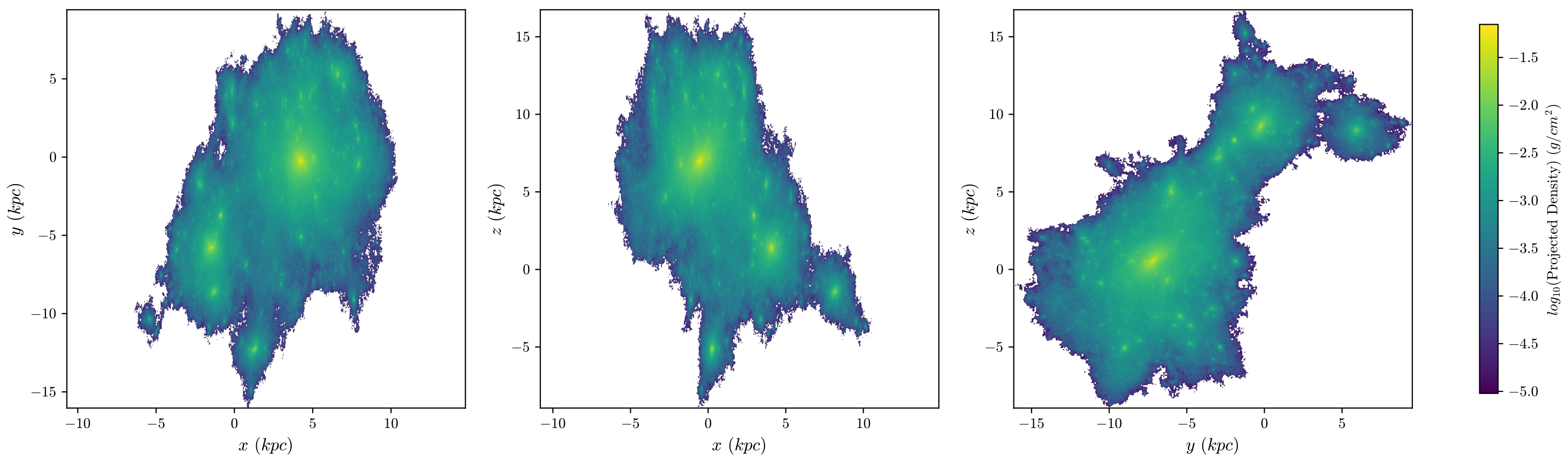
halo8 Stars, z = 3.027 , 512 bins
