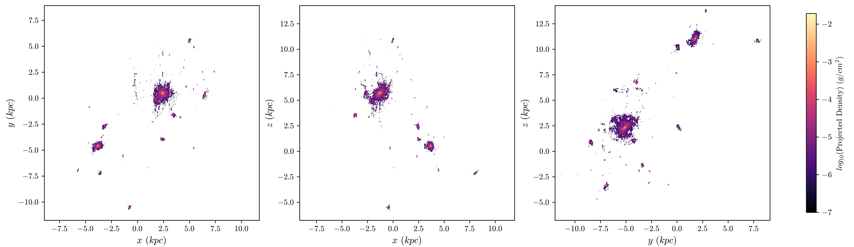
halo8 Stars, z = 3.027 , 512 bins
