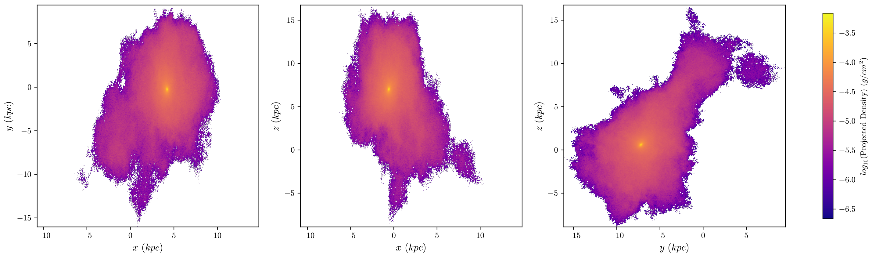
halo8 Dark Matter, z = 3.027 , 512 bins
