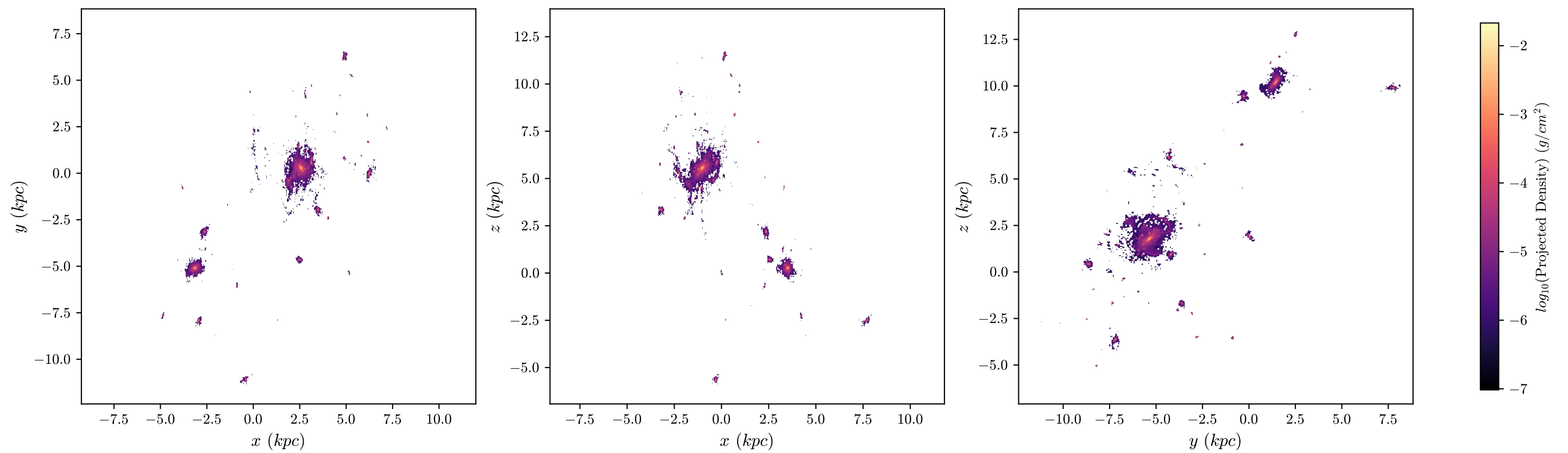
halo8 Stars, z = 3.008 , 512 bins
