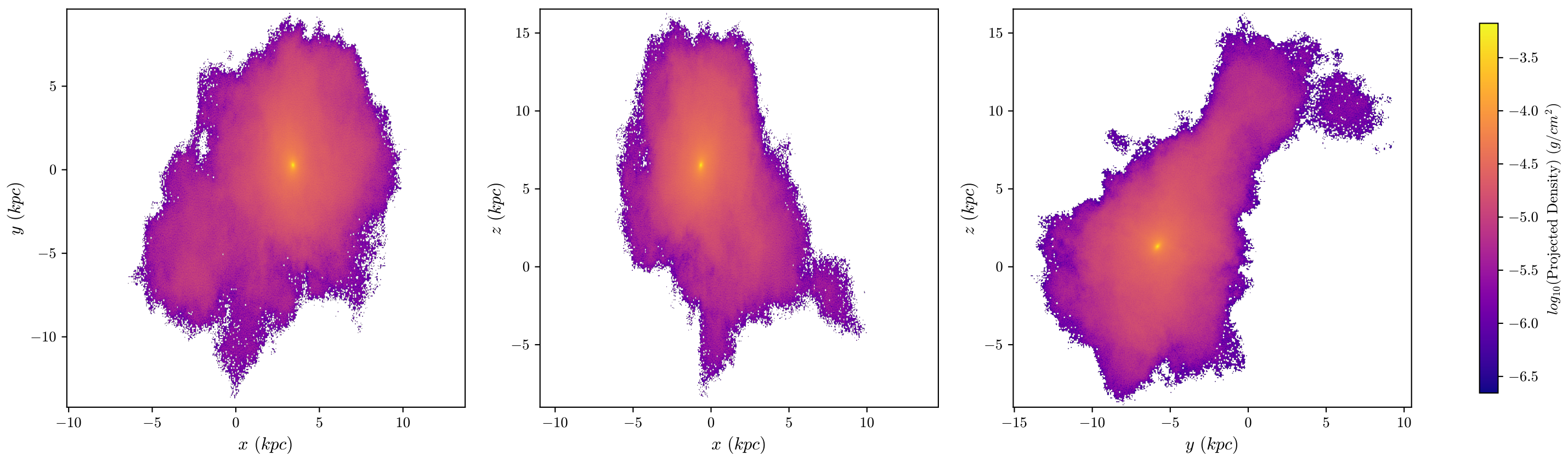
halo8 Dark Matter, z = 3.008 , 512 bins
