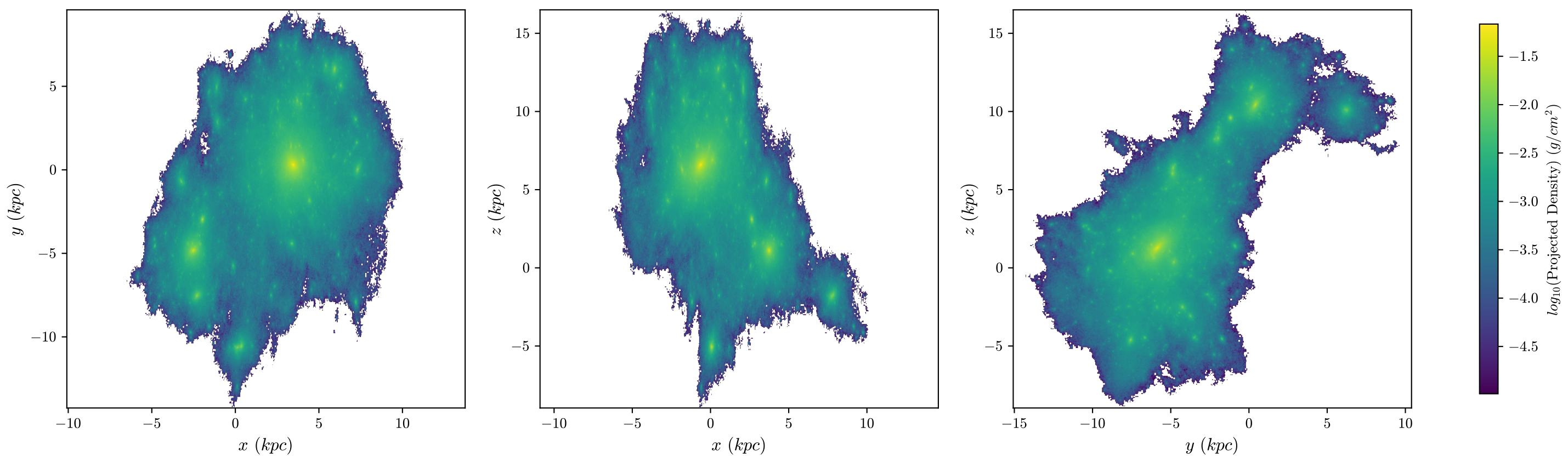
halo8 Stars, z = 3.008 , 512 bins
